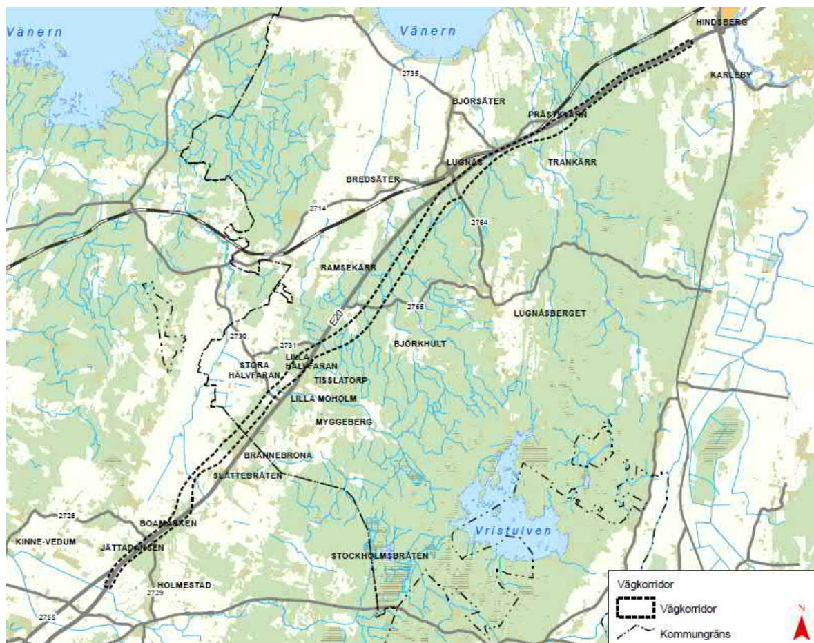
Figur 2.6.1 Geografisk avgränsning. Svart streckad linje är vald vägkorridor (Blå/Grön) för E20, det utgör även miljökonsekvensbeskrivningens huvudsakliga geografiska avgränsning.
