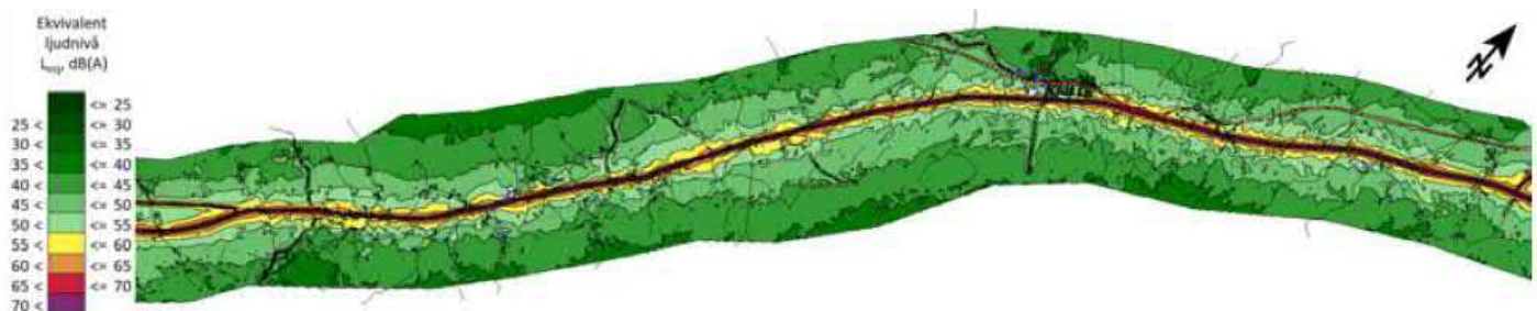
Figur 3.5.6.3 Nollalternativ, ekvivalent ljudnivå två meters höjd samt bostäder.
