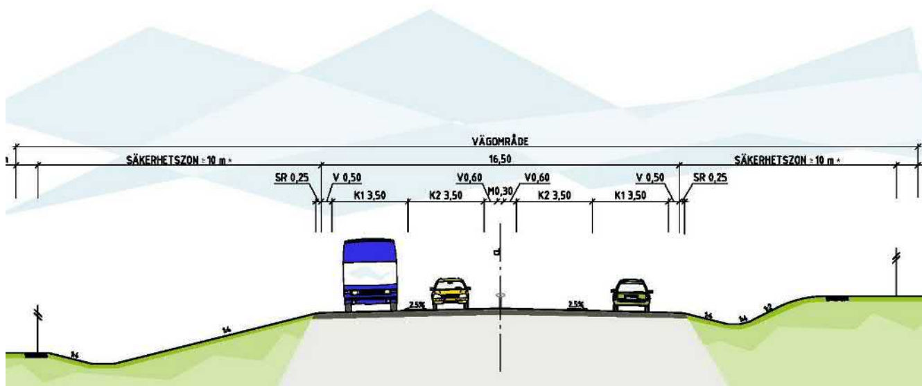
Figur 4.2.1.2 Typsektion E20 med 2+2 körfält.
