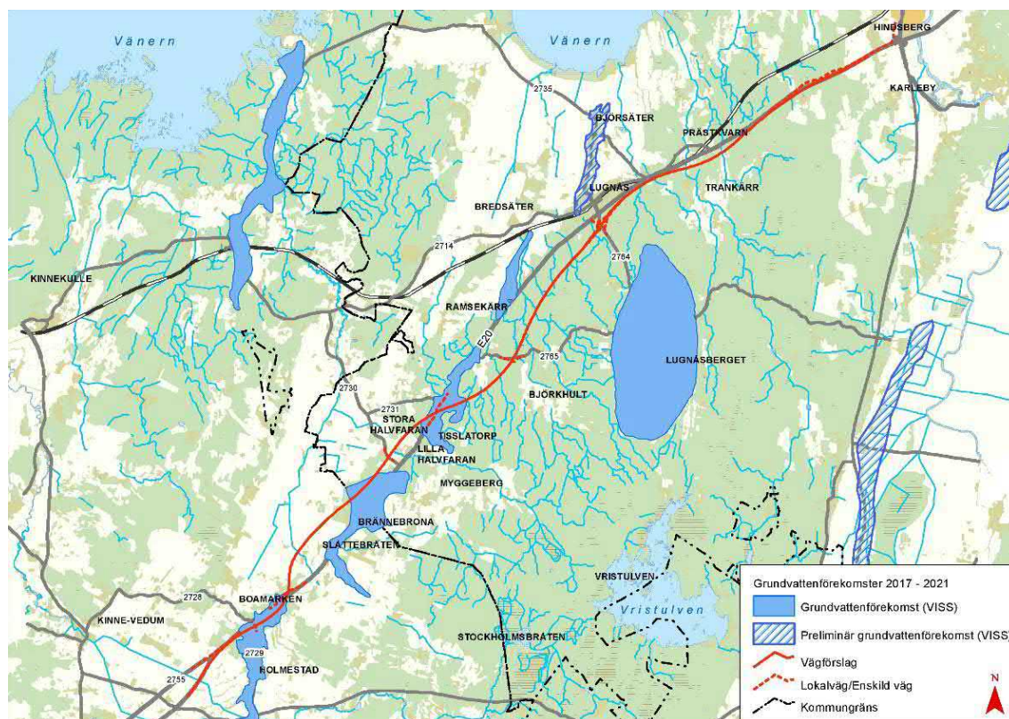
Figur 3.6.2.3 Grundvattenförekomster i området.
