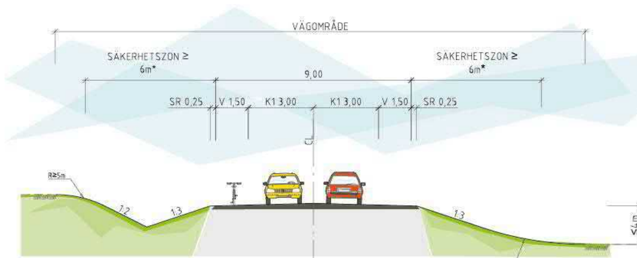
Figur 4.2.1.4 Typsektion lokalväg 2755.
