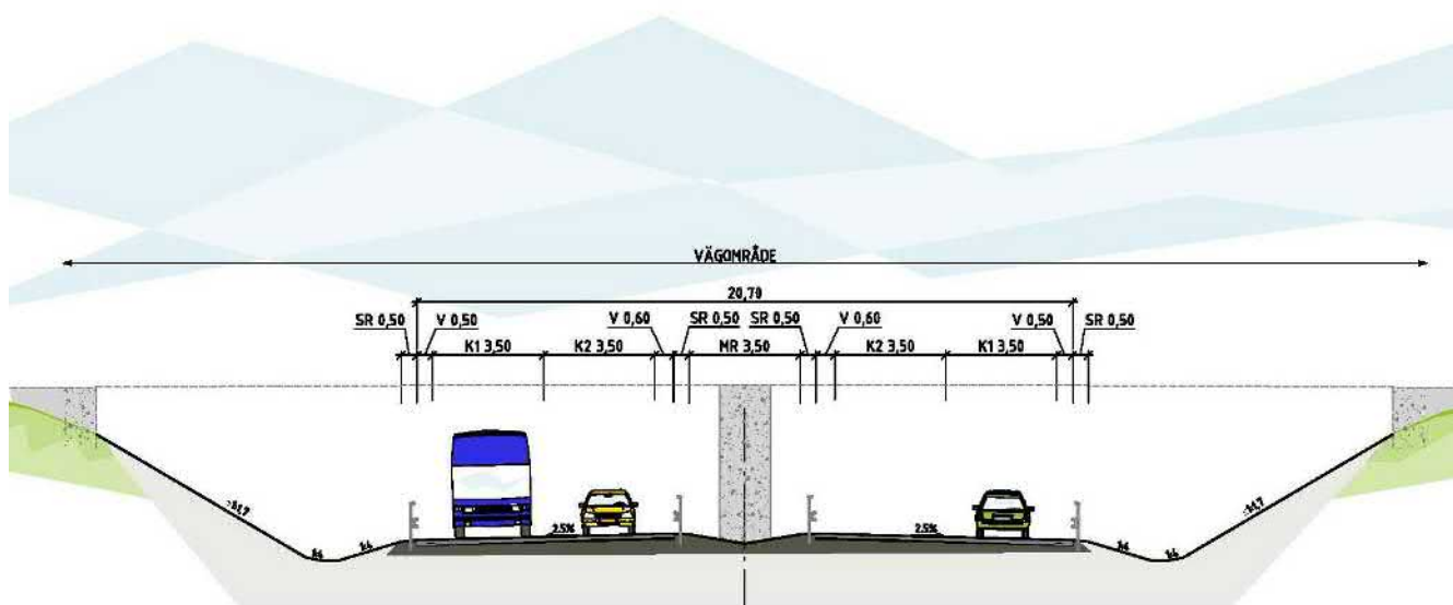
Figur 4.2.1.3 Typsektion E20 och bro över med 2+2 körfält.
