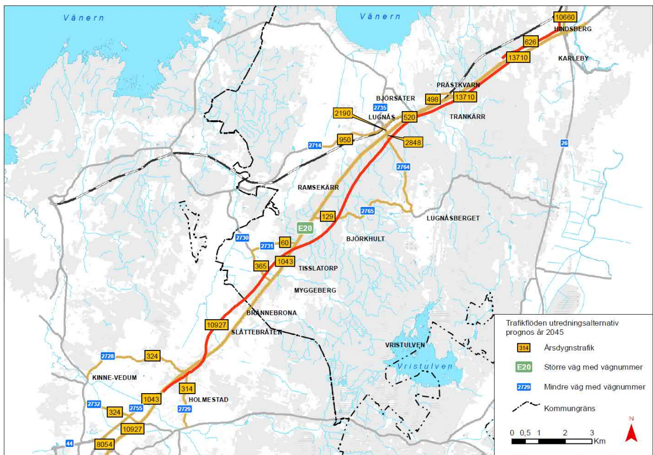
Figur 5.1.1.1 Trafikflöden i utredningsvägnätet, totaltrafik, ÅDT prognosår 2045.
