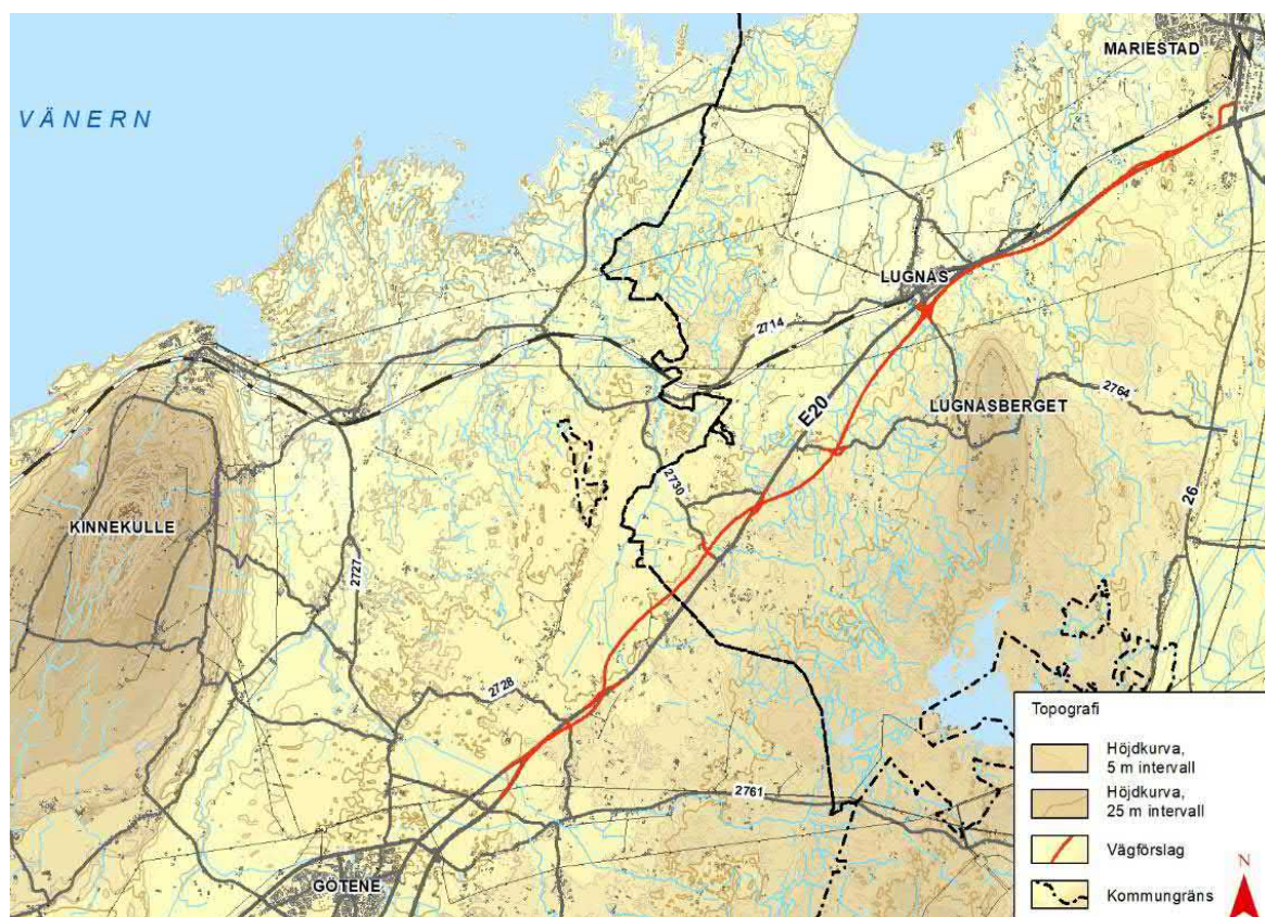
Figur 3.5.2.1 Områdets topografi. De större strukturerna i landskapet löper i sydvästlig-nordöstlig sträckning. E20 har samma riktning och ligger i övergångszonen mellan högsta och lägsta kustlinjen, mellan moränområdena i öster och slätterna i väster.
