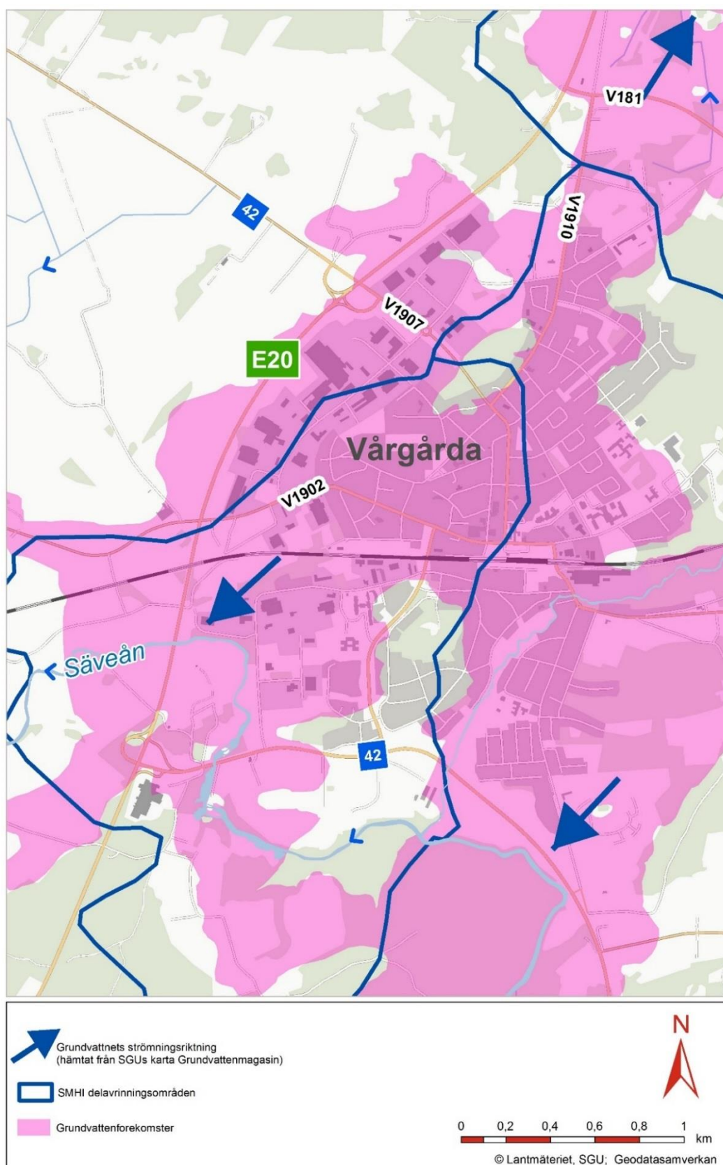
Figur 17 - Grundvattenförekomst, Säveån och vattendelare samt bedömd strömningsriktning grundvatten.
