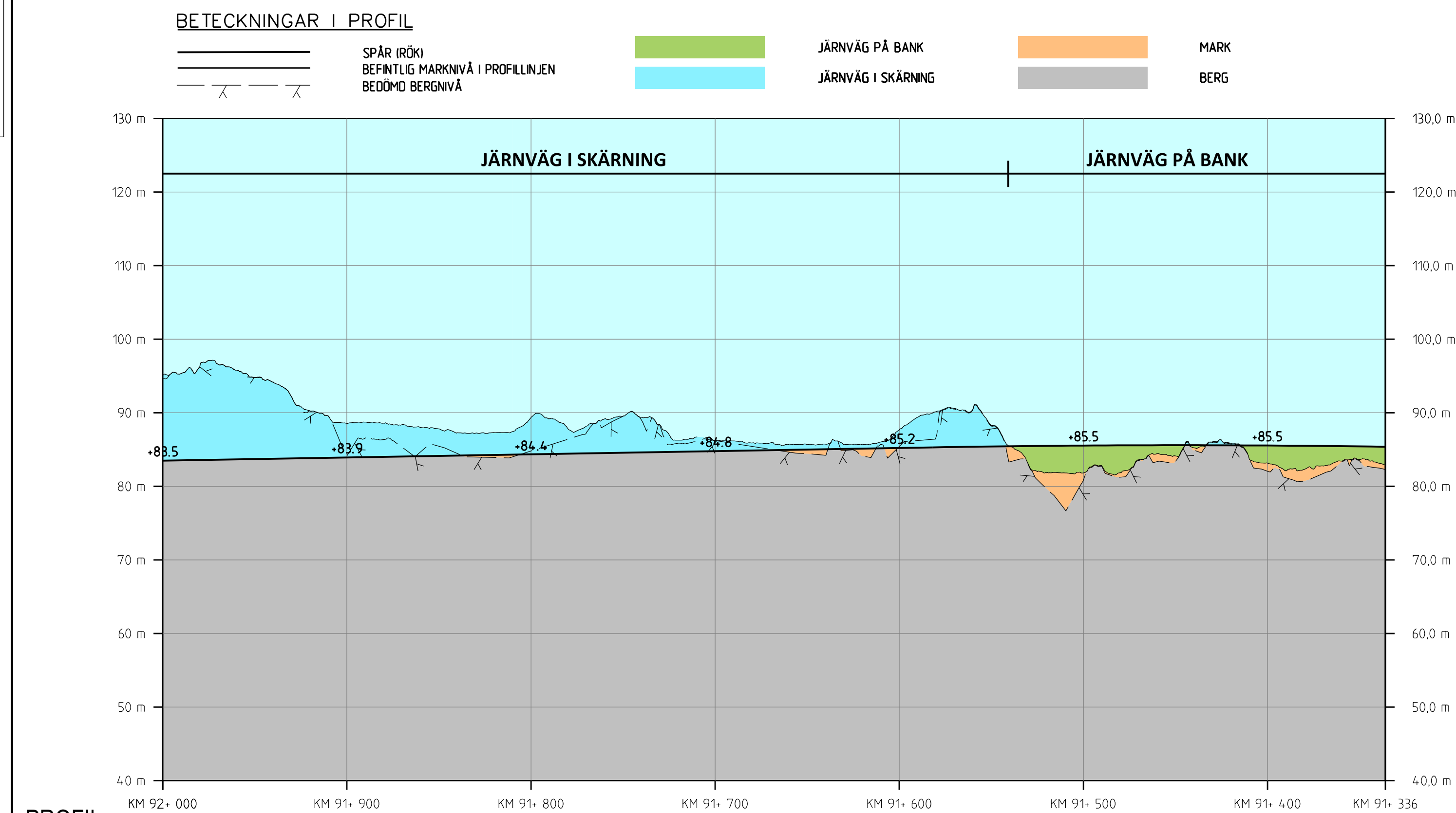
PROFIL SPÅRPROFIL LÄNGS NEDSPÅRET (ÖSTLIGA SPÅRET)
