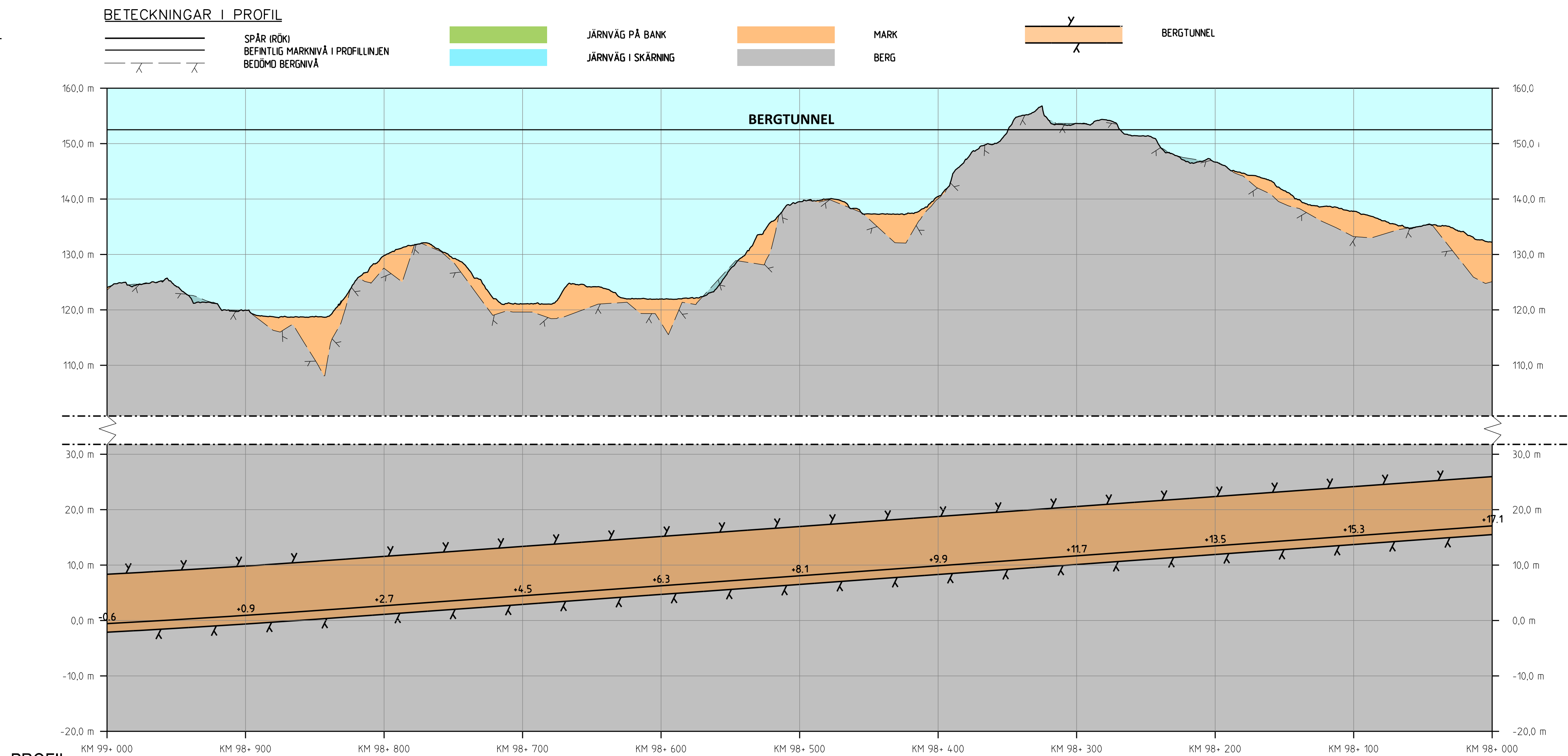
PROFIL SPÅRPROFIL LÄNGS NEDSPÅRET (ÖSTLIGA SPÅRET)
