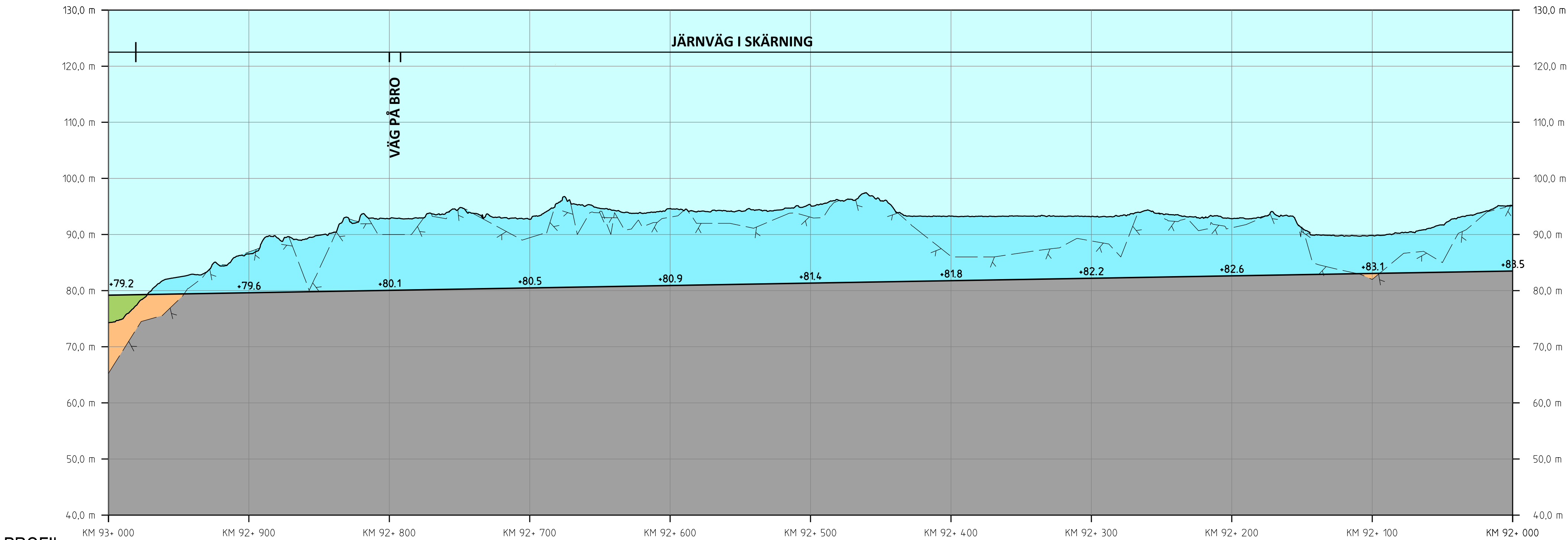
PROFIL SPÅRPROFIL LÅNGS NEDSPÅRET (ÖSTLIGA SPÅRET)
