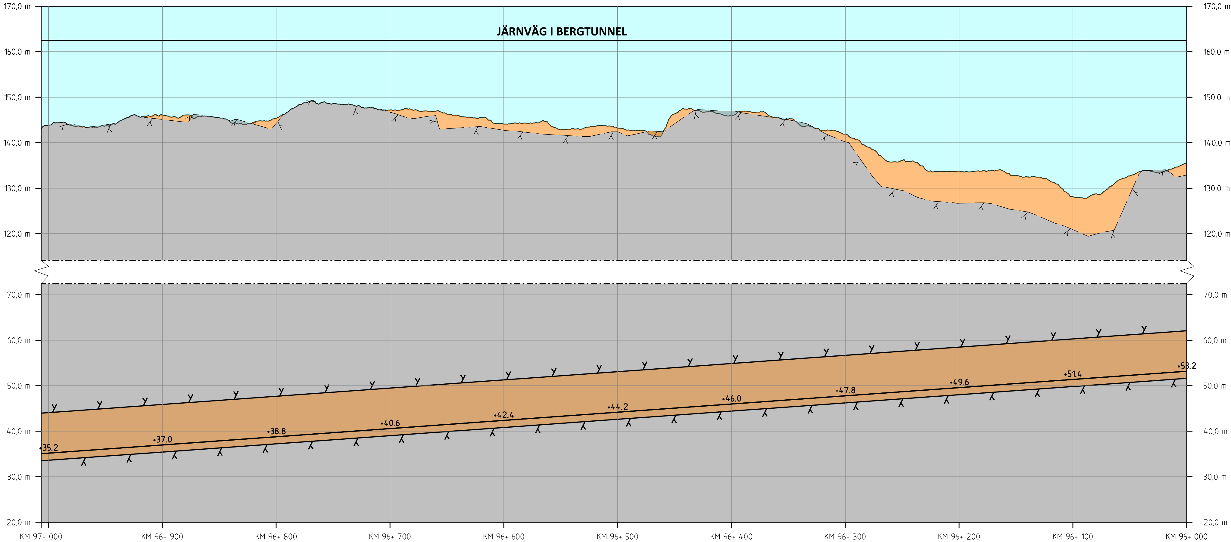
PROFIL SPÅRPROFIL LÅNGS NEDSPÅRET (ÖSTLIGA SPÅRET)
