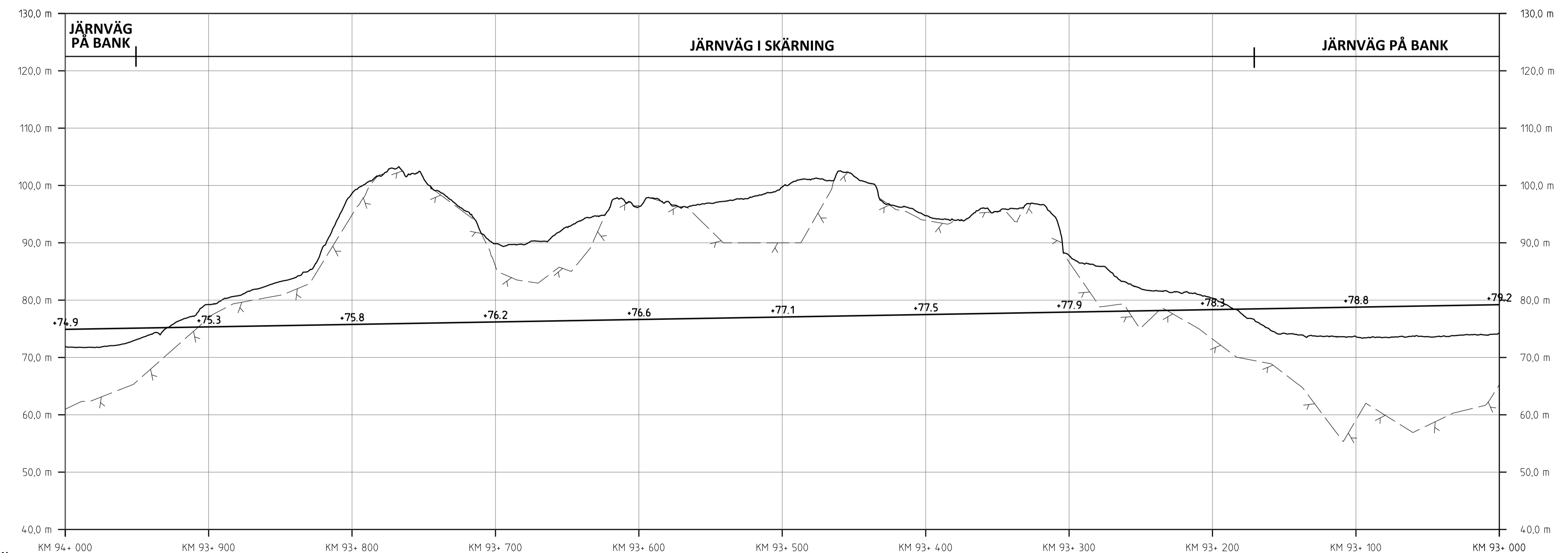
PROFIL SPÄRPROFIL LÄNGS NEDSPÅRET (ÖSTLIGA SPÅRET)
