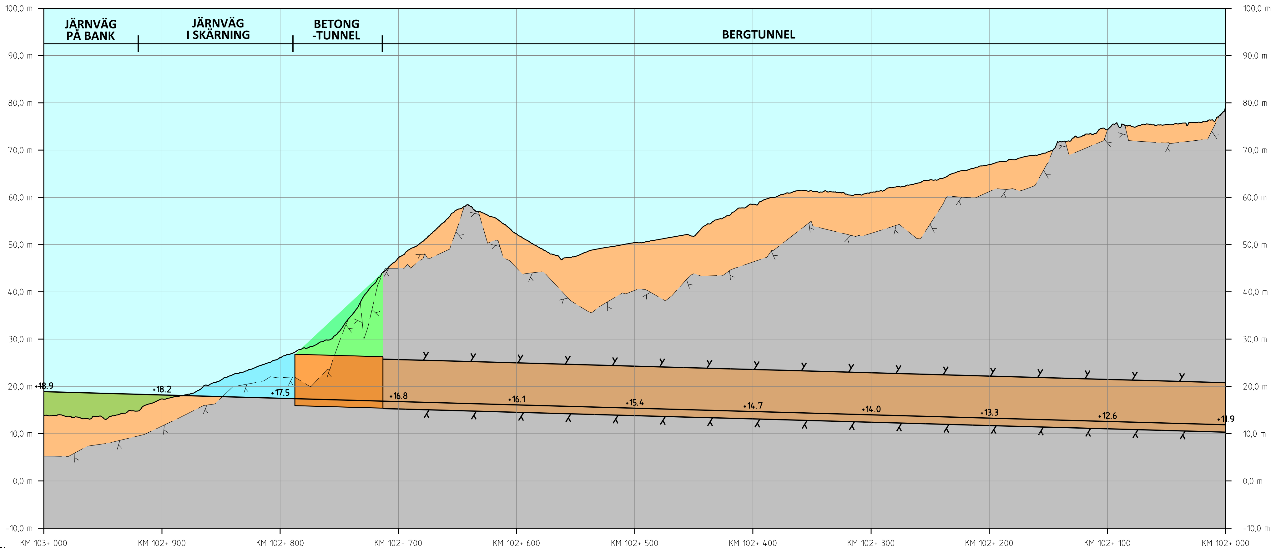
PROFIL SPÅRPROFIL LÄNGS NEDSPÅRET (ÖSTLIGA SPÅRET)
