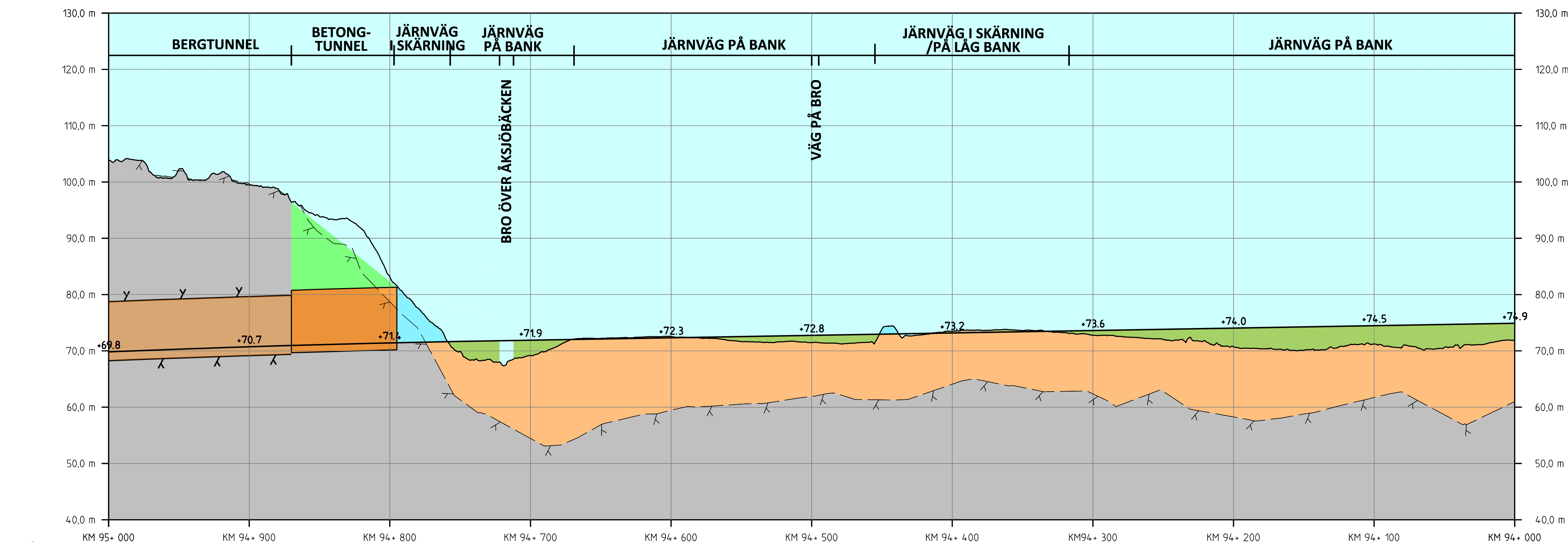
PROFIL SPÄRPROFIL LÄNGS NEDSPÄRET (ÖSTLIGA SPÄRET)
