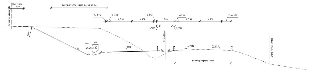
Figur 7. Typsektion ytväg 2+2 körfält med mitträcke vid breddning av befintlig väg (Tpl Gladö- Tpl Slätmossen).
