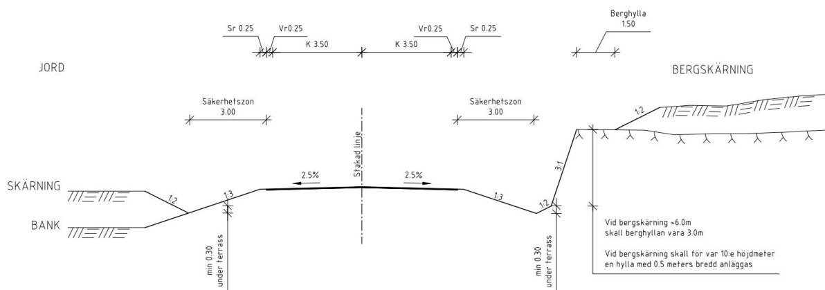
Figur 51. Typsektion lokalväg.
