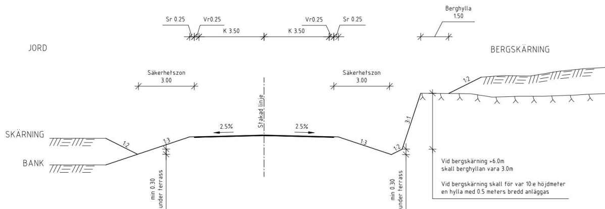
Figur 48. Typsektion lokalväg.
