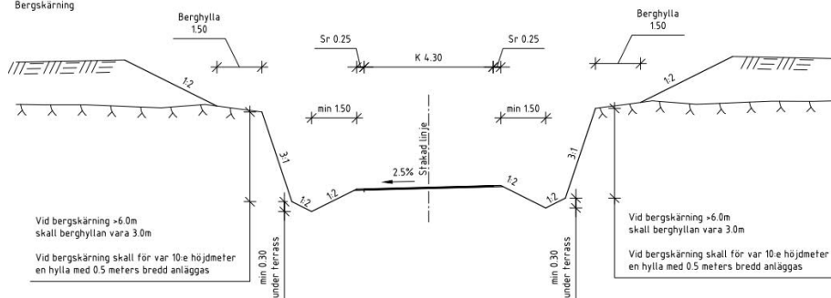
Figur 33 Typsektion gång- och cykelväg bergskärning
