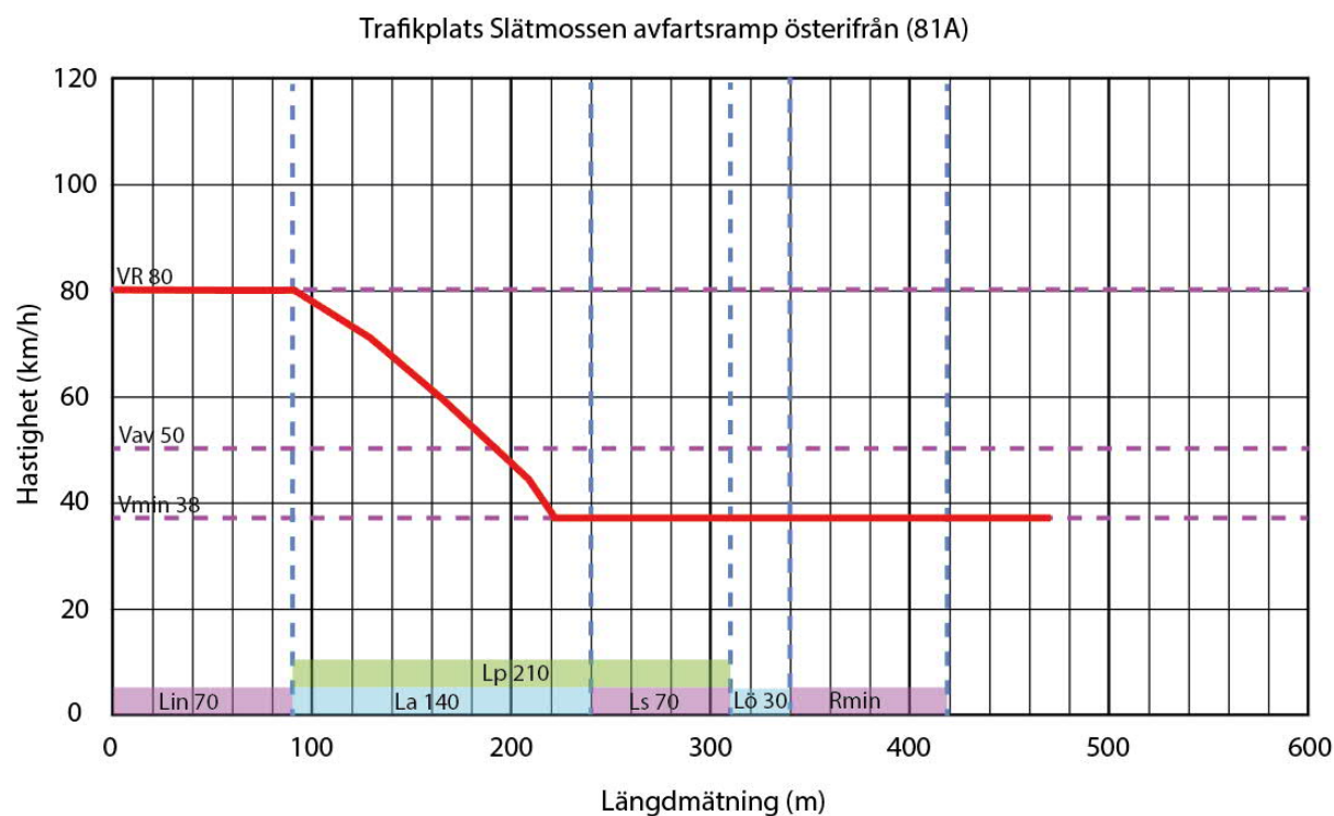
Figur 74 Hastighetsprofil avseende personbil (Pb) för trafikplats Slätmosse, avfart österifrån
