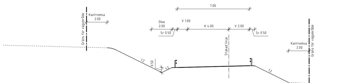
Figur 50. Typsektion för ramp ytväg.
