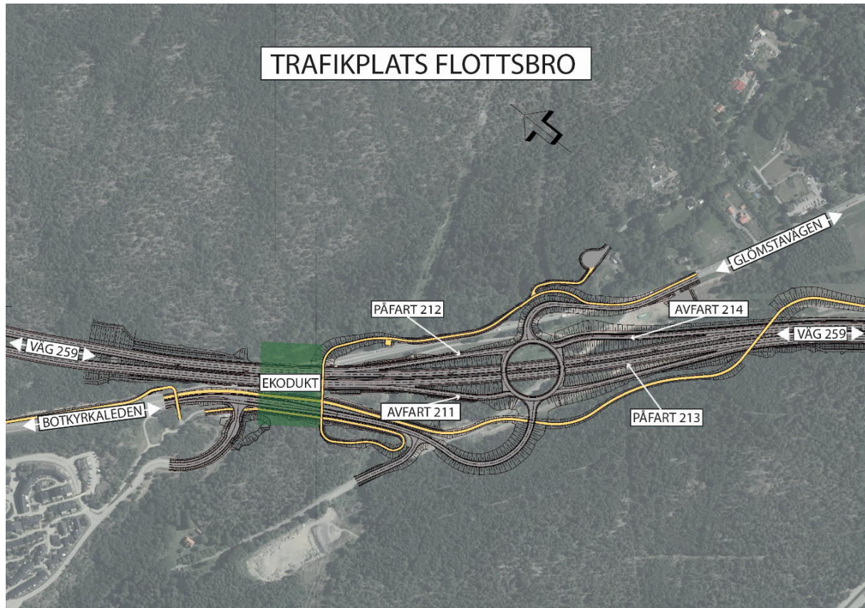
Figur 46. Trafikplats Flottsbro.
