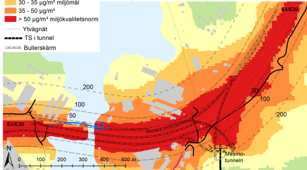
Figur 2. Beräknade dygnsmedelhalter av partiklar, PM10 ( \mu\text{g}/\text{m}^3 ) under det 36:e värsta dygnet i utbyggnadsalternativ år 2045 visas som halvfält. Överskrider halten 50 \mu\text{g}/\text{m}^3 överskrider miljökvalitetsnormen. Är halten högre än 30 \mu\text{g}/\text{m}^3 uppnås inte miljömålet. Streckade linjer visar avstånd från Tvärförbindelsen för 50, 100 och 200 meter. Gråa ytor motsvarar befintlig bebyggelse. Från SLB 10:2019.
