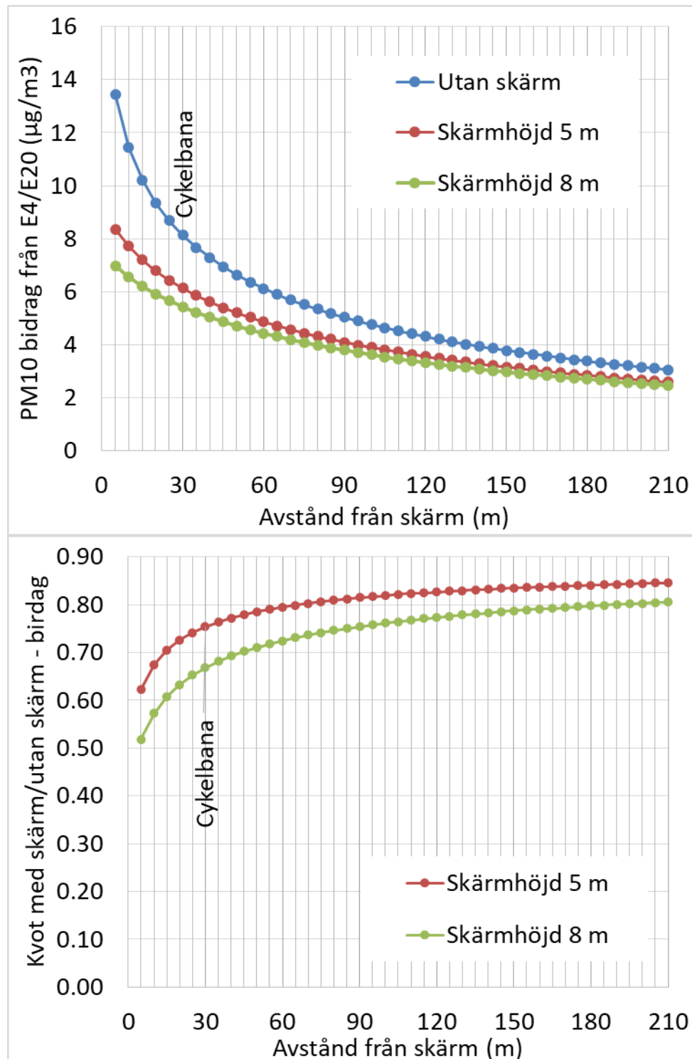
Figur 19. Beräknade bidrag till PM10 halterna (årsmedelvärden) utan skärm, med 5 & 8 meter hög skärm (övre diagrammet) samt kvoten mellan halterna med skärm och utan skärm (undre diagrammet). Värden gäller för tvärsnittet som definieras med den prickade linjen i Figur 17.
