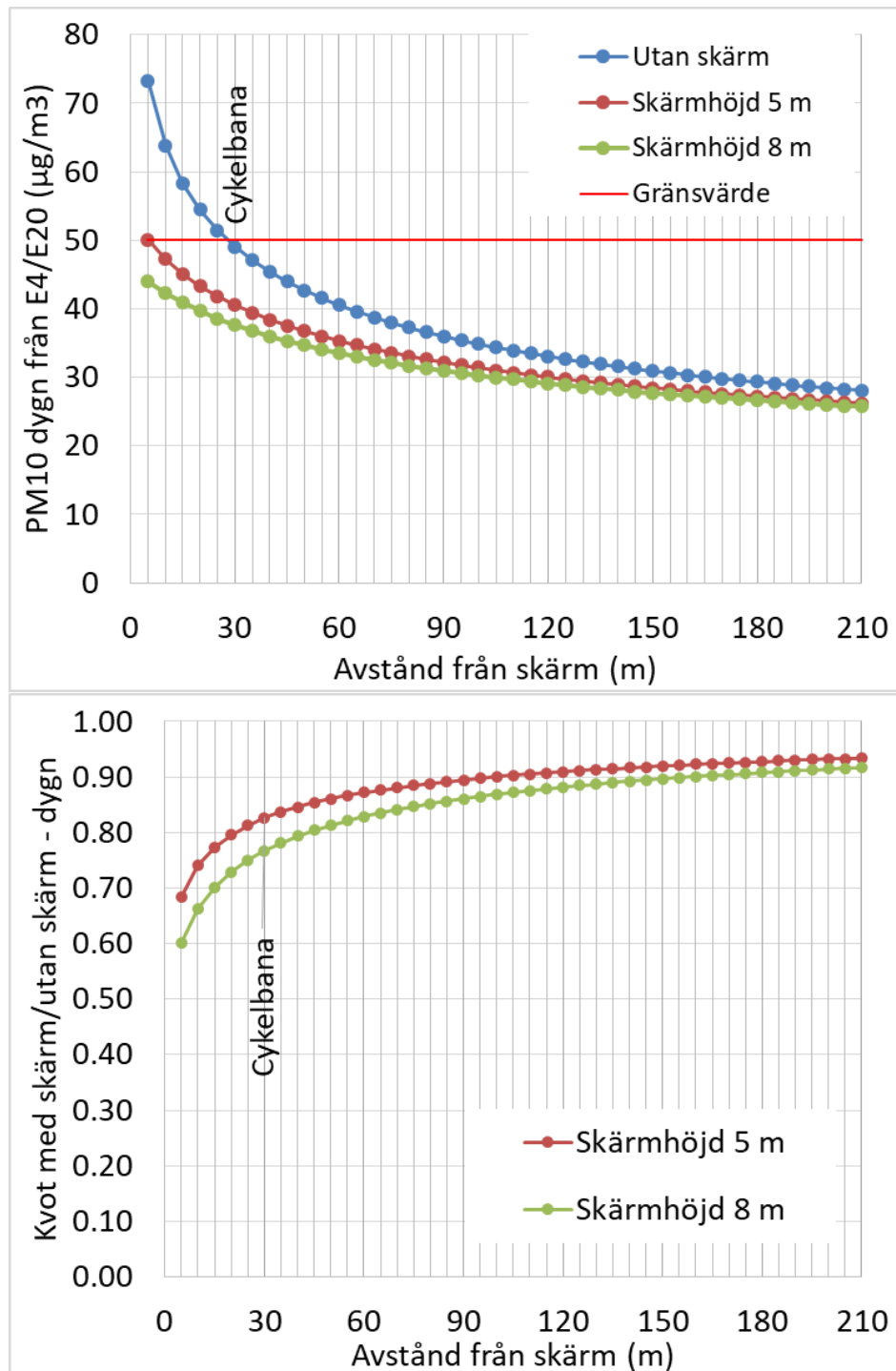
Figur 20. Beräknade totala PM10 halterna (36:e högsta dygnsmedelvärdet) utan skärm, med 5 & 8 meter hög skärm (övre diagrammet) samt kvoten mellan halterna med skärm och utan skärm (undre diagrammet). Värden gäller för tvärsnittet som definieras med den prickade linjen i Figur 17.
