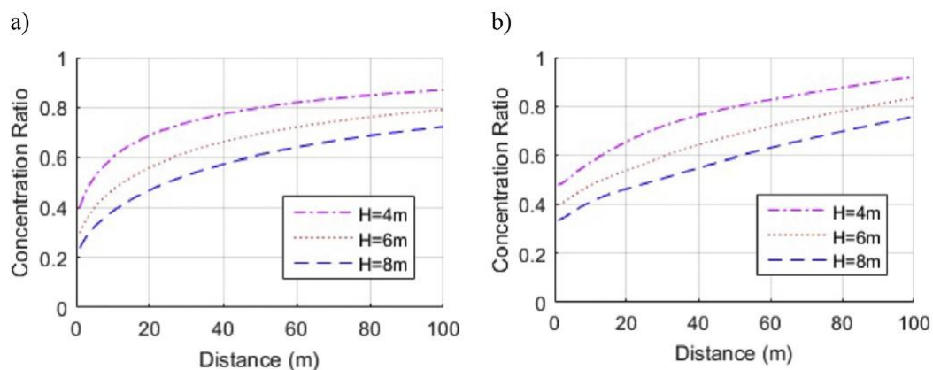
Figur 16. Koncentration med skärm i förhållande till utan skärm på olika avstånd från en skärm som är 4, 6 och 8 meter hög. Beräkningar med respektive utan hänsyn till om luften är instabilt skiktad (b) eller neutralt skiktad (a), enligt Amini et al. (2016).
