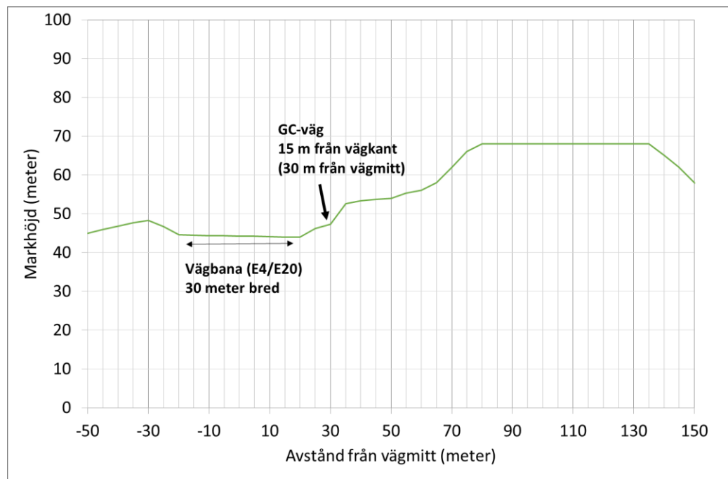
Figur 18. Topografin i tvärsnittet markerat med prickad linje i Figur 17.
