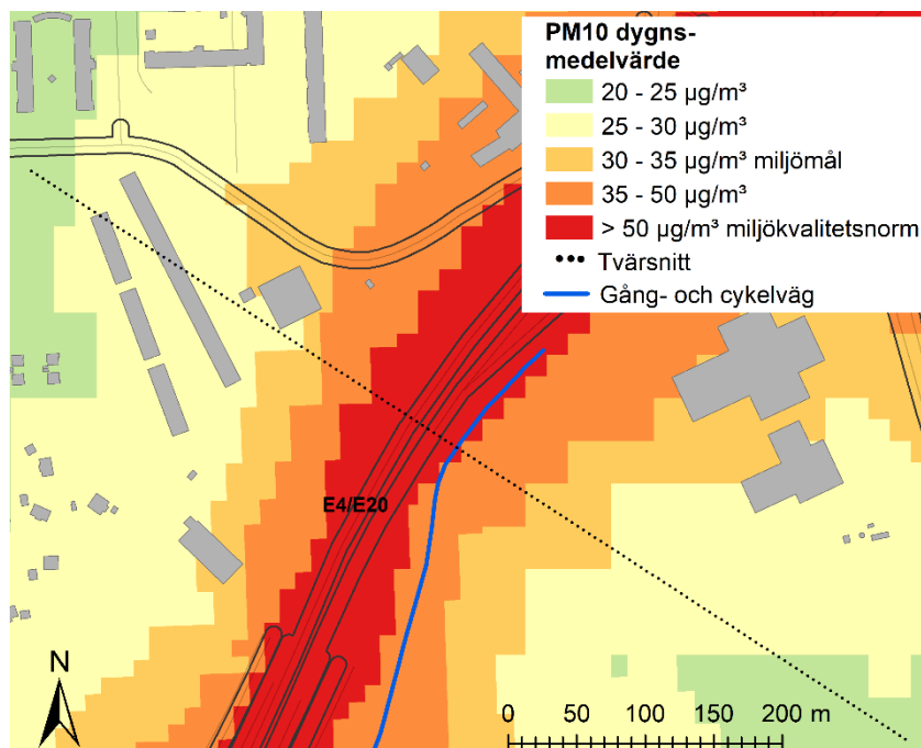
Figur 17. PM10 halter (36:e högsta dygnsmedelvärde) i anslutning till E4/E20 vid Vårby backe med Tvärförbindelse Södertörn år 2045. Halter över 50 \mu\text{g}/\text{m}^3 innebär att miljökvalitetsnormen överskrids. Halten högre än 30 \mu\text{g}/\text{m}^3 innebär att miljömålet överskrids. Gråa ytor motsvarar befintlig bebyggelse. Prickade linjen visar tvärsnittet som använts för beräkningarna av bullerskärmens betydelse.
