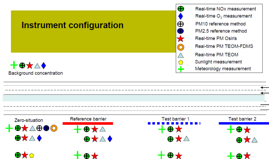
Figur 11. Mätstationer och mätinstrument i studien av Hooghwerff et al. (2010).
