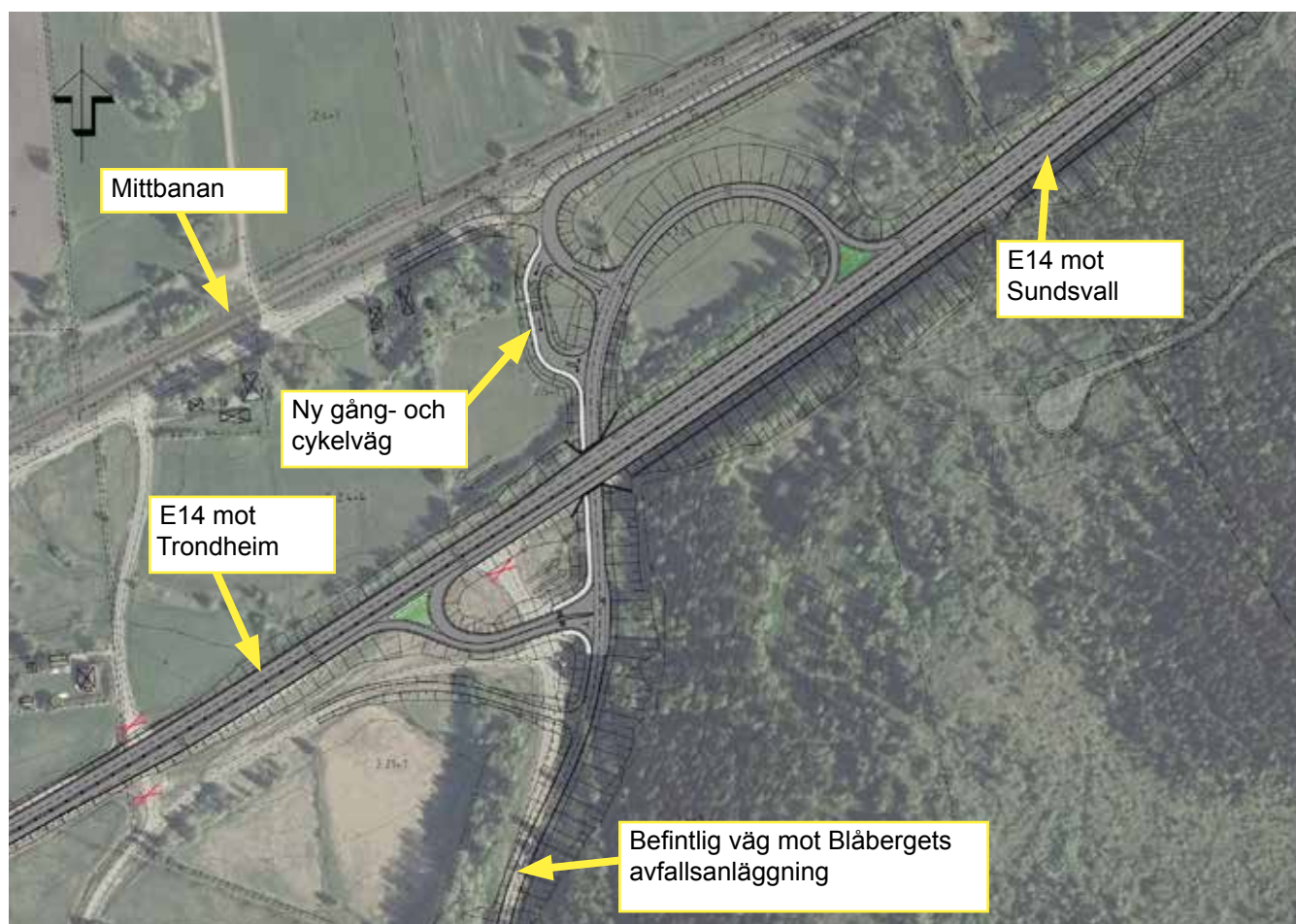
Figur 3.2:1 Planskild anslutning vid Blåberget.
