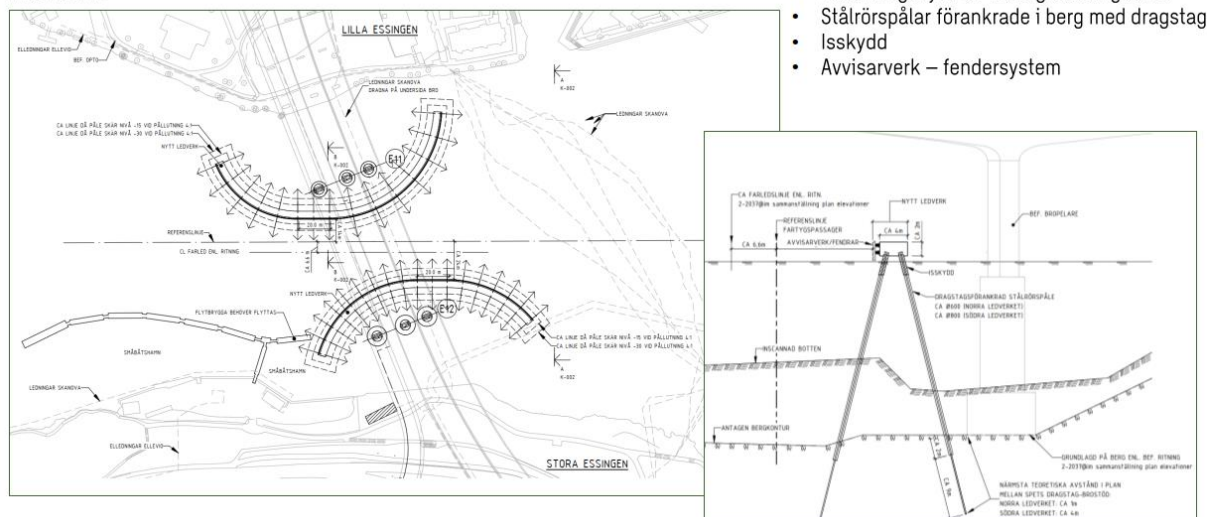
Figur 2. Skissförslag för valt alternativ från PM Byggnadsverk
