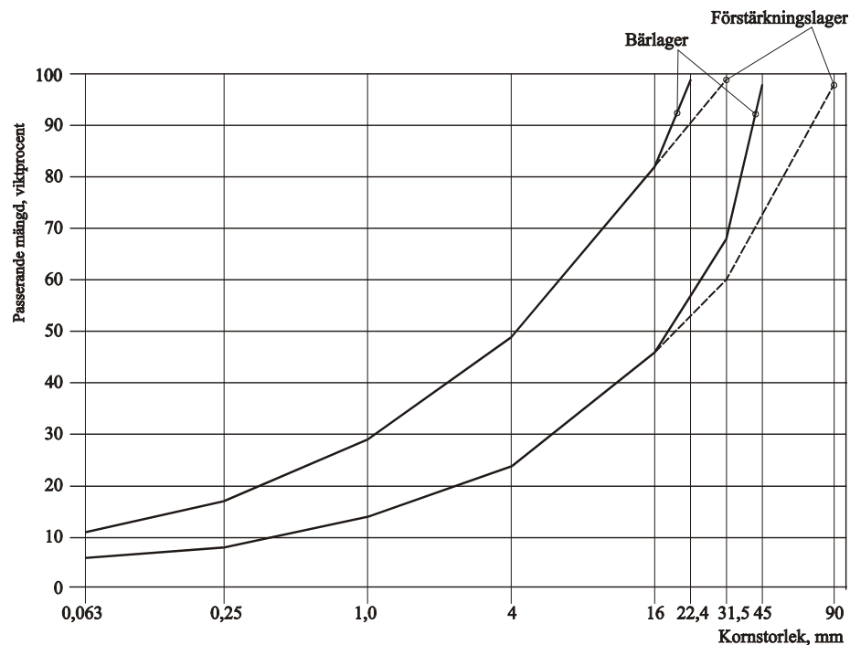
Figur B6.3-2 Illustration av materialets kornstorleksfördelning för bärlager och förstärkningslager i grusväg.
