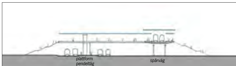
Solvalla plan och sektion A-A. Utformningsförslag där stationsbyggnad läggs på bro mellan spårväg och pendeltågsplattformar.
