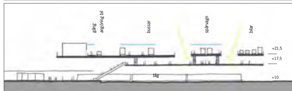
Barkarby Stockholm Väst plan och sektion A-A. I detta förslag läggs stationen på vägbro över järnvägen.
