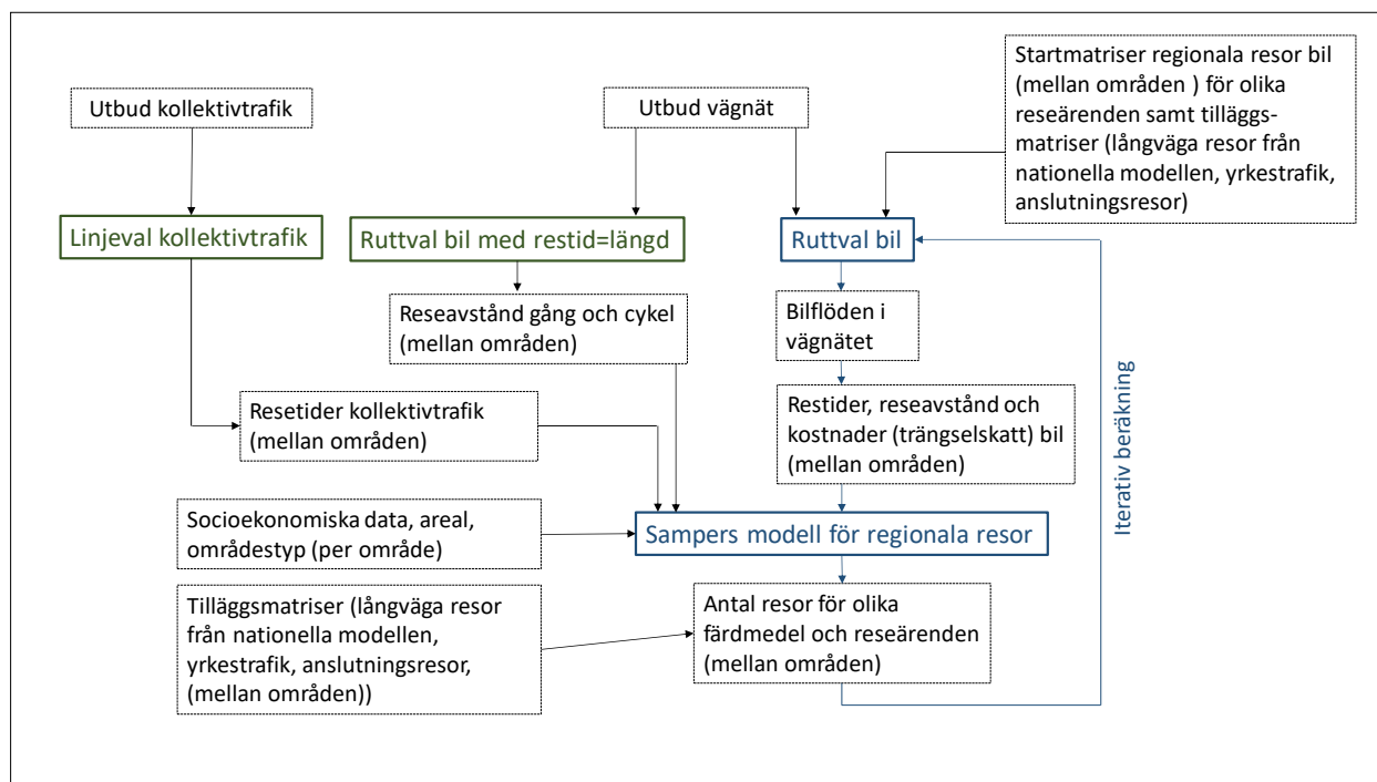
Figur 3: Schematisk beskrivning av beräkningsprocessen för trafikprognoser för regionala resor i Utbud JA (och Utbud UA).
