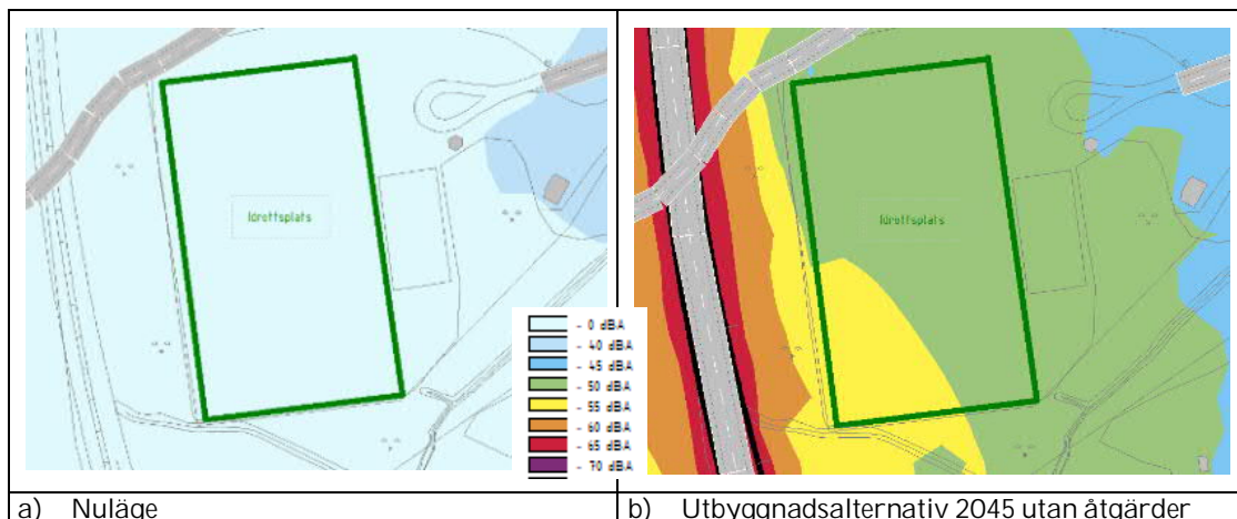
Figur 11. Ekvivalent ljudnivå 2 m över mark, idrottsplats.
