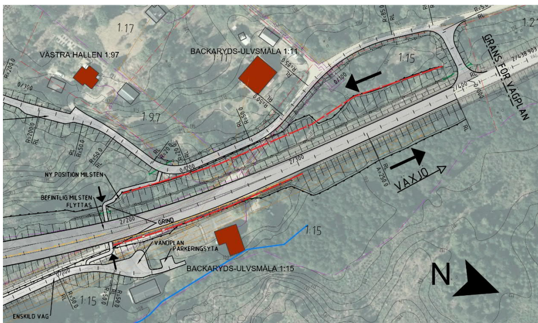
Figur 4. Möjligt läge för vägnära bullerskydd i vägplanens norra del, markerade med röd färg. Bullerberörda byggnader markerade med brun färg.
