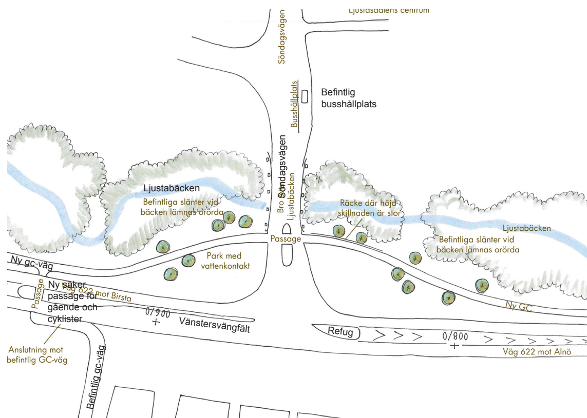
Figur 5.8 Illustration visande korsningen med Söndagsvägen. Gång- och cykelvägen följer Ljustabäcken och svänger in mot centrumbebyggelsen i Ljustadalen. Avståndet mellan gång- och cykelvägen och väg 622 behövs för trafiksäkerheten i korsningen. En parkliknande yta skapas som dessutom ger en mer vilsam miljö för de gående.
