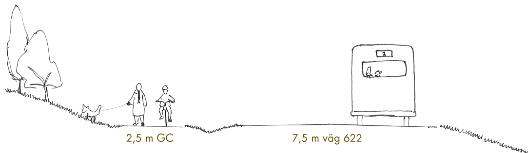
Figur 5.1 Illustration visande hur väg och gångväg förhåller sig till varandra där gång- och cykelvägen ligger separerad från väg 622. De separeras av ett flackt dike sått med gräs. Dikets bredd är 3 meter.
