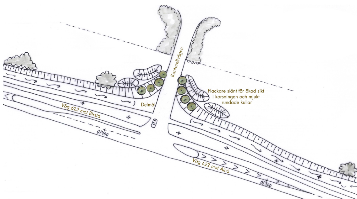
Figur 5.6 Illustration visande korsningen med Kantarellvägen. En ny trädrad markerar infarten till bostadsområdet. Tillsammans med det nya vänstersvängfältet gör den korsningen tydligare och säkrare. Korsningen blir också ett delmål för dem som nyttjar gång- och cykelvägen.
