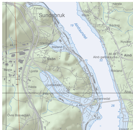
Figur 4.12. Standnivåkartan visar den forntida fördelningen mellan hav och land. För 2000 år utgjordes den nuvarande dalgången av en djup havsvik. Karta Sveriges geologiska undersökning (SGU).
