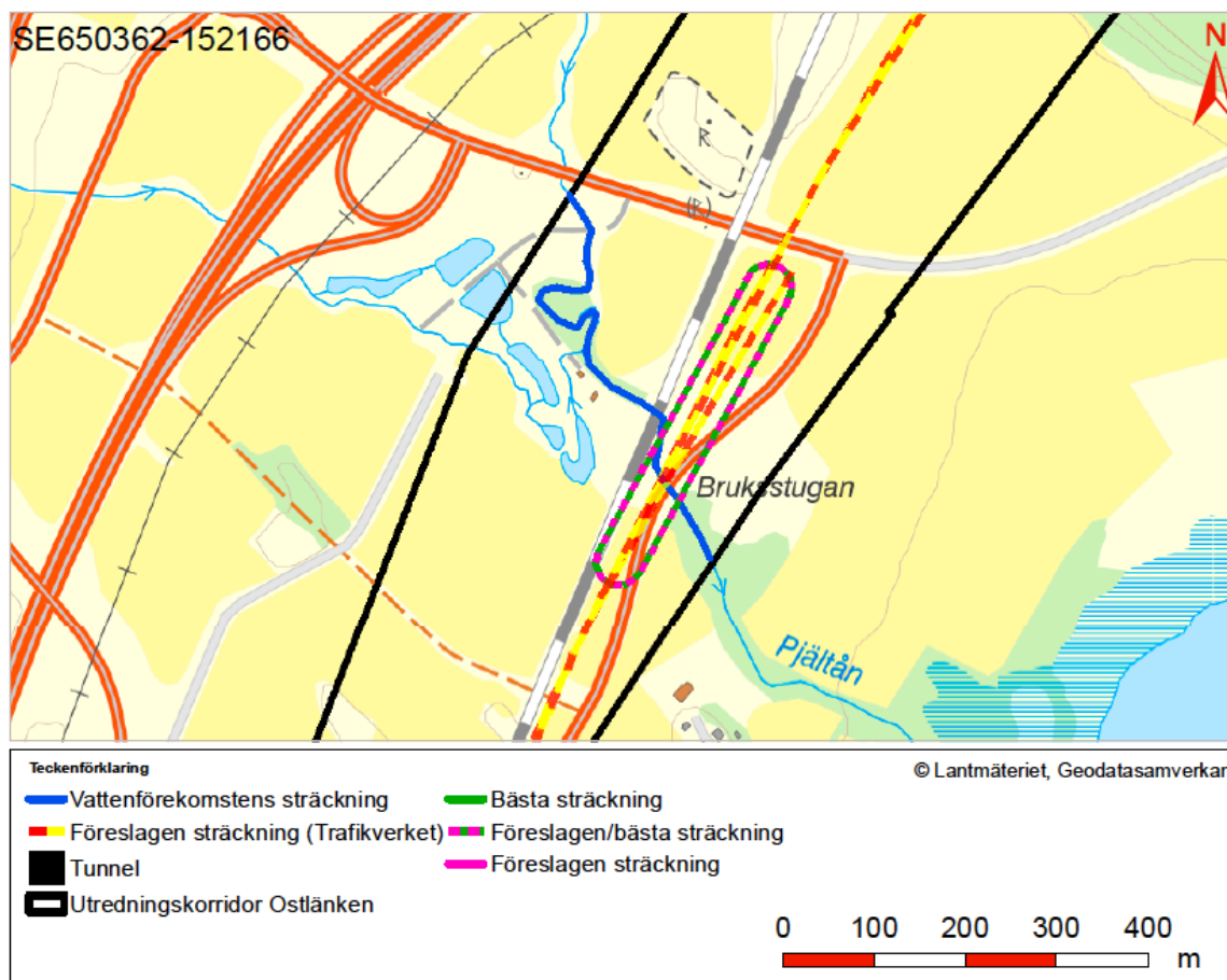
Figur 8. Förslagen sträckning vid korsningarna med Pjältån.
