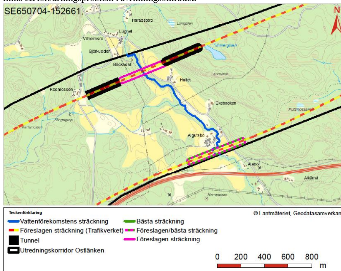
Figur 4. De två alternativa förslagen till sträckning vid Getåbäcken. Påverkansområdena är små vid båda förslagen till sträckning. Inget av alternativen bedöms påverka ekologisk eller kemisk status.
