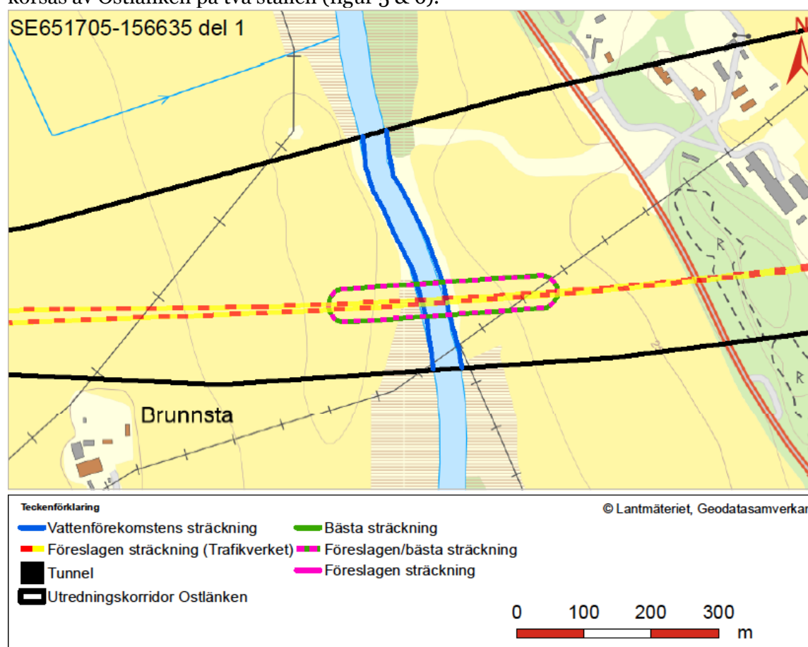
Figur 5. Föreslagen sträckning vid en av korsningarna med Nyköpingsån.
