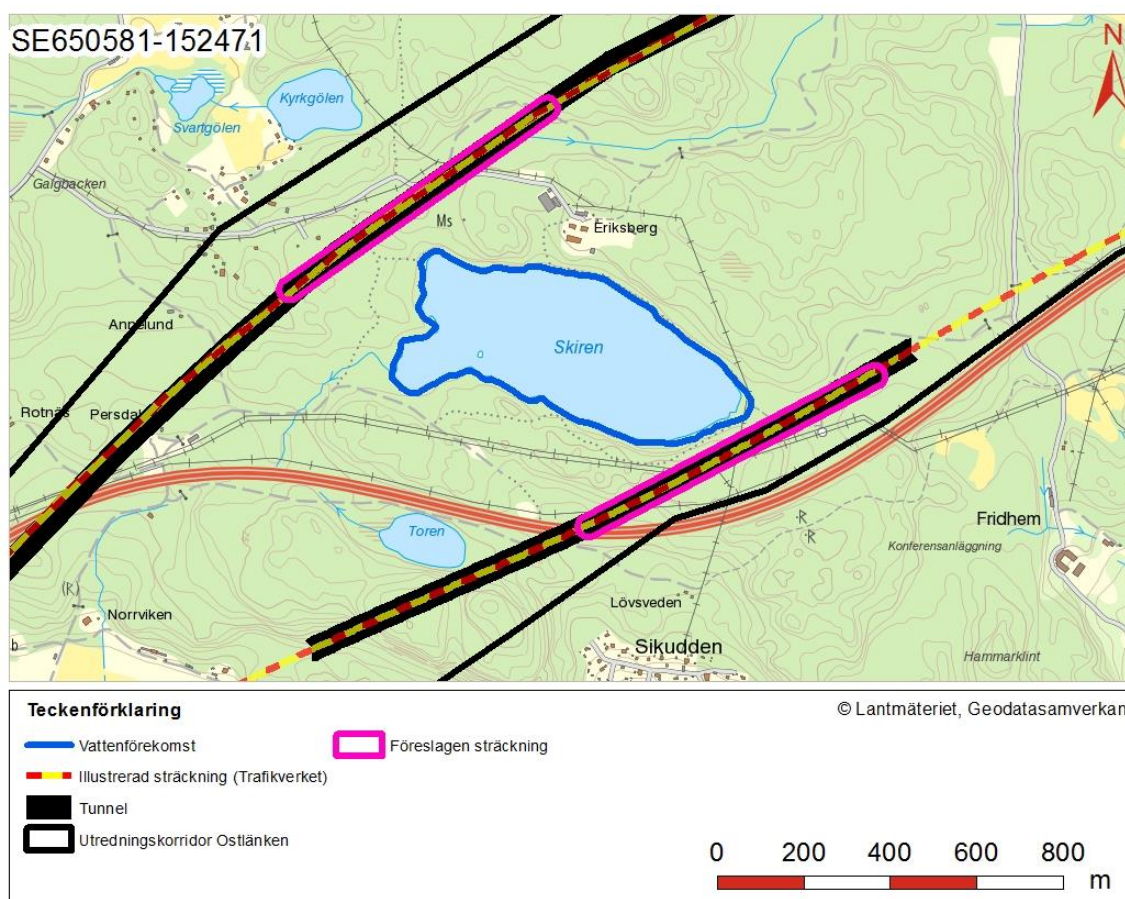
Figur 11. Kartan illustrerar de två alternativa dragningarna som Trafikverket föreslagit.
