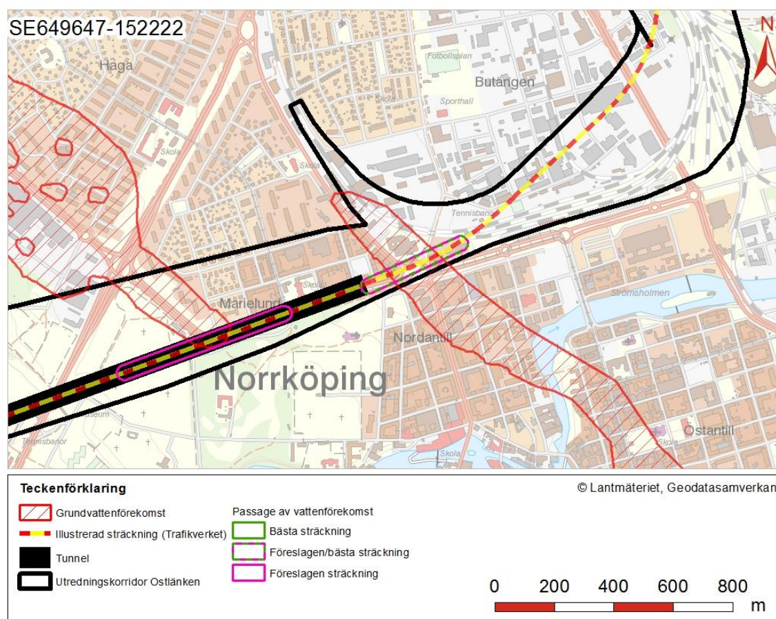
Figur 16. Kartan illustrerar Trafikverkets planerade sträckning.
