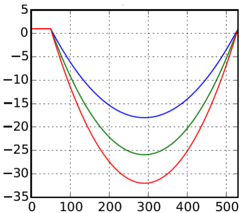
Figur 29. Illustration från utredning år 2016 över vajerns form när linfärjan ligger still vid Larshamn, Yxlan.
