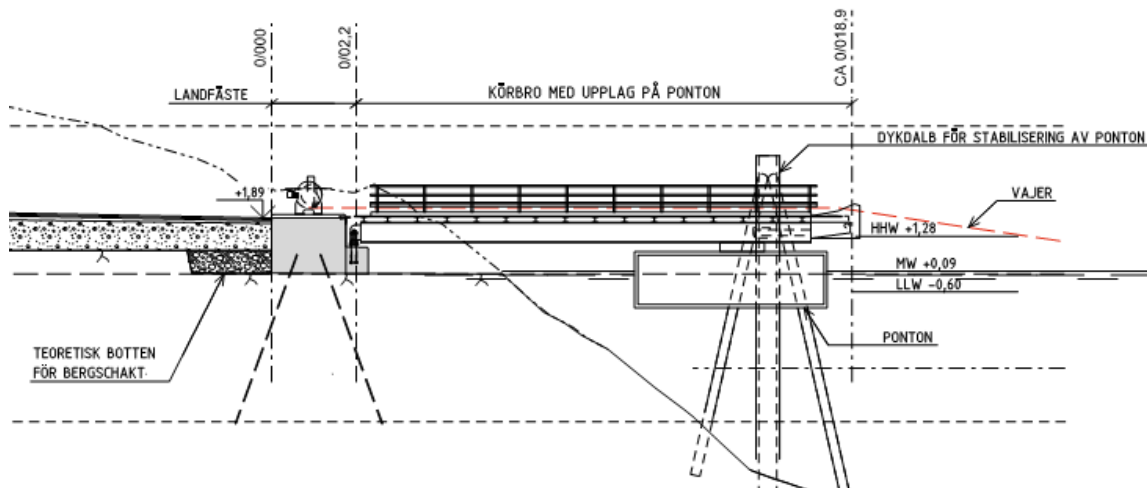
Figur 27. Typsektion av pontonläge.
