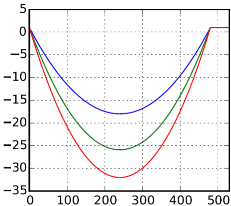
Figur 30. Illustration från utredning år 2016 över vajerns form när linfärjan ligger still vid Norrsund, Blidö.
