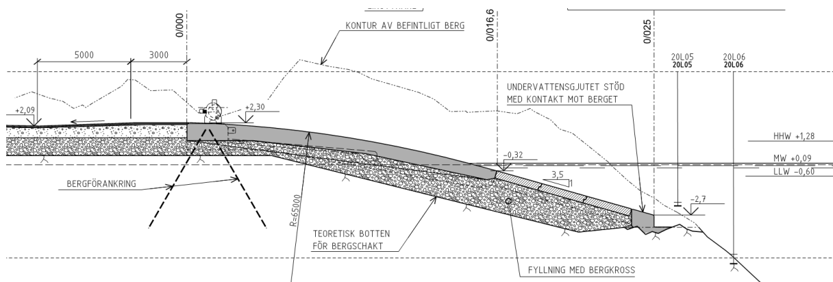
Figur 26. Typsektion av betongramp.
