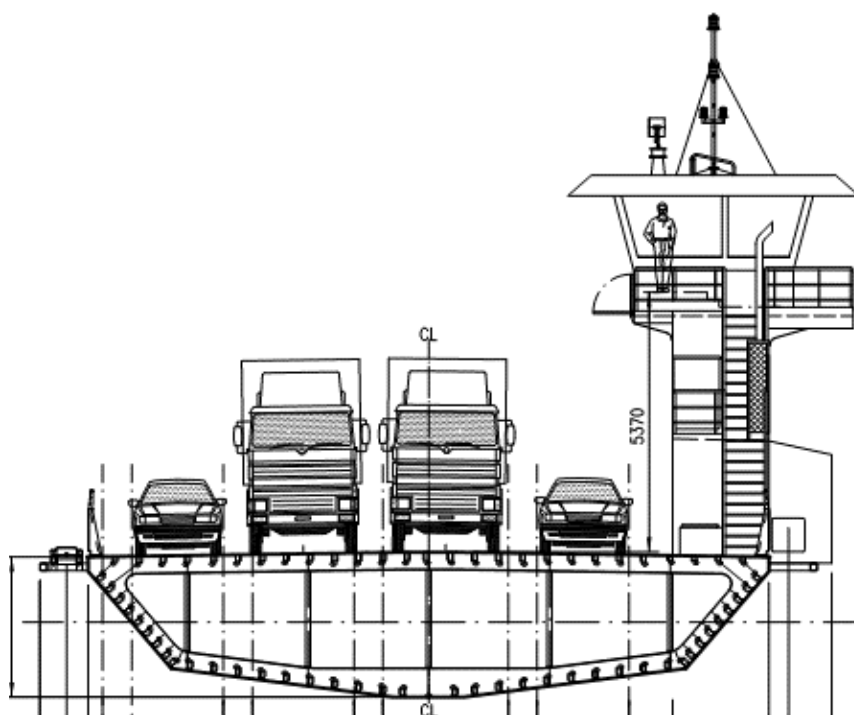
Figur 15. Tvärs­ek­tion av linfärja
