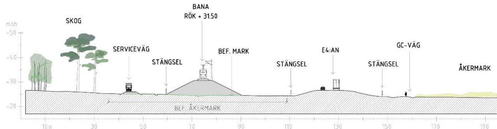
Figur 4.3-5 Järnvägens utformning vid Täfteåns mosaiklandskap.
