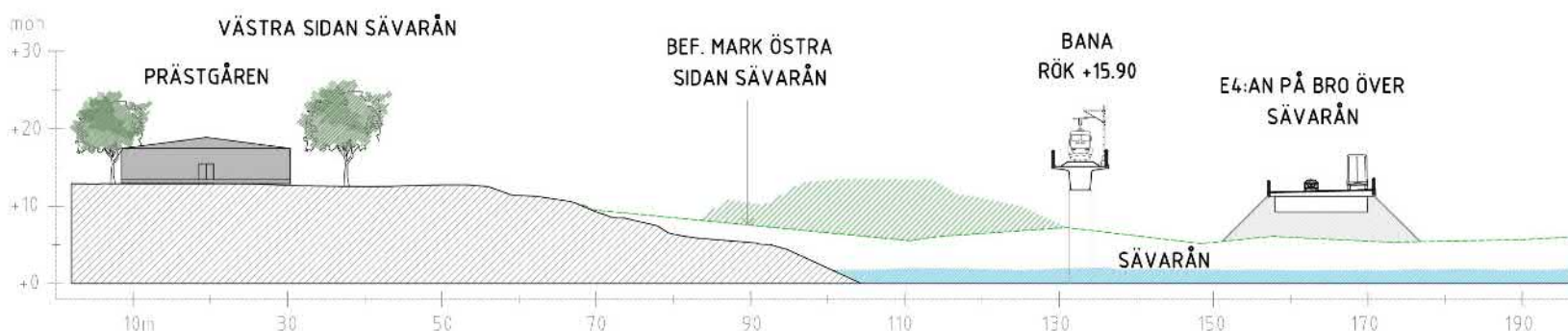
Figur 4.3-7 Järnvägens passage över Sävarån.
