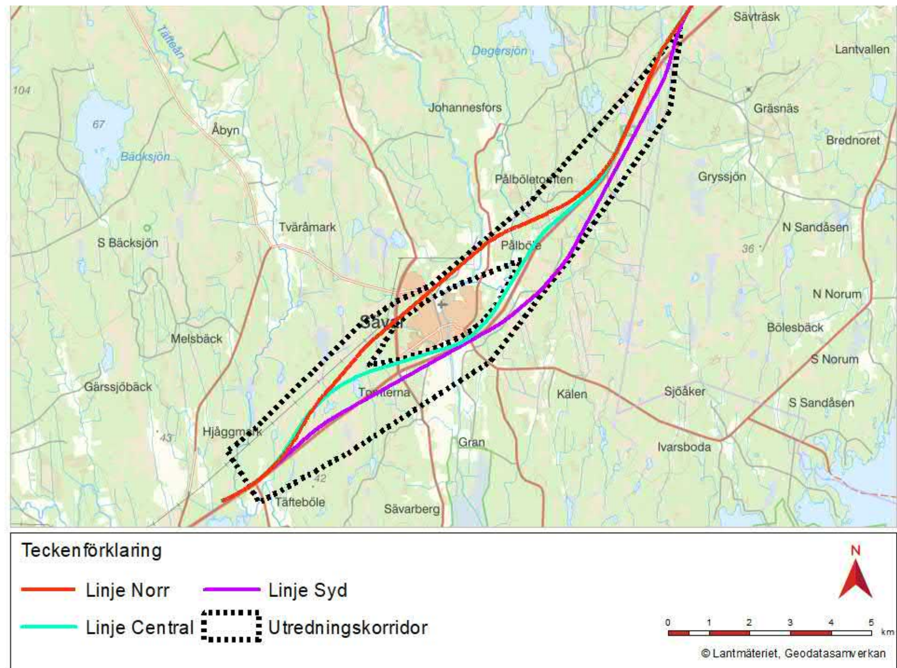
Figur 4.2-2. Kvarstående alternativ efter fördjupade linjestudier på sträckan Däva-Gryssjön.
