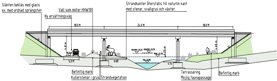
Figur 4.3-10 Sektion av järnvägsbro över Täfteån, km 12+475.
