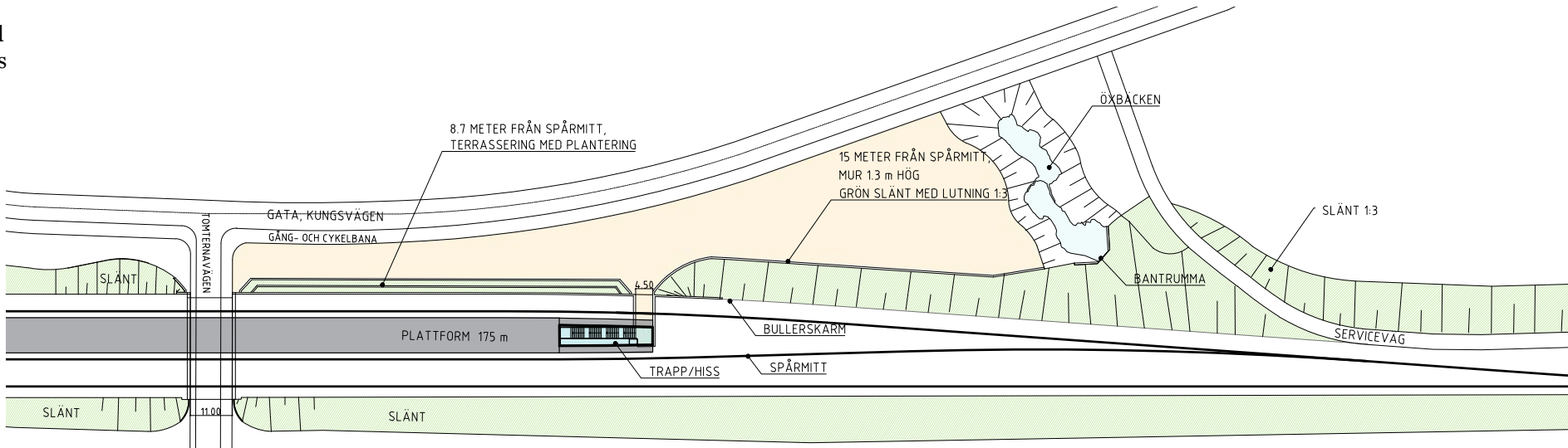
Figur 4.3-4 Förslag på utformning av regionaltågsstationen i Sävar.
