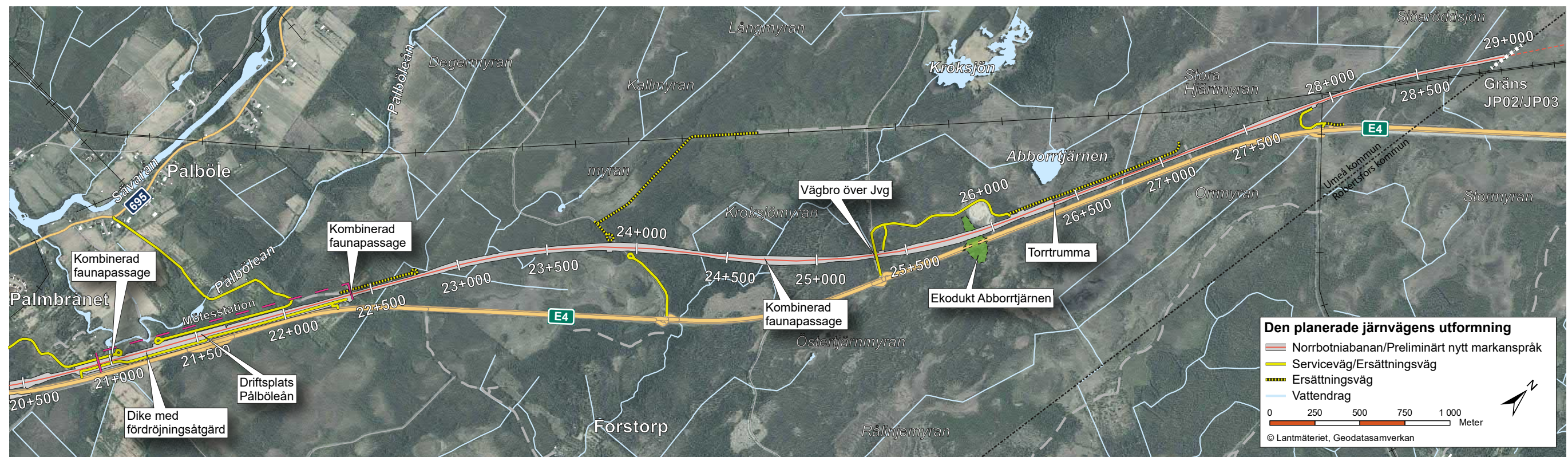
Figur 4.3-2. Översiktskarta över delsträckan Däva-Gryssjön som visar den norra delen av Norrbotniabananans sträckning med planerad utformning.
