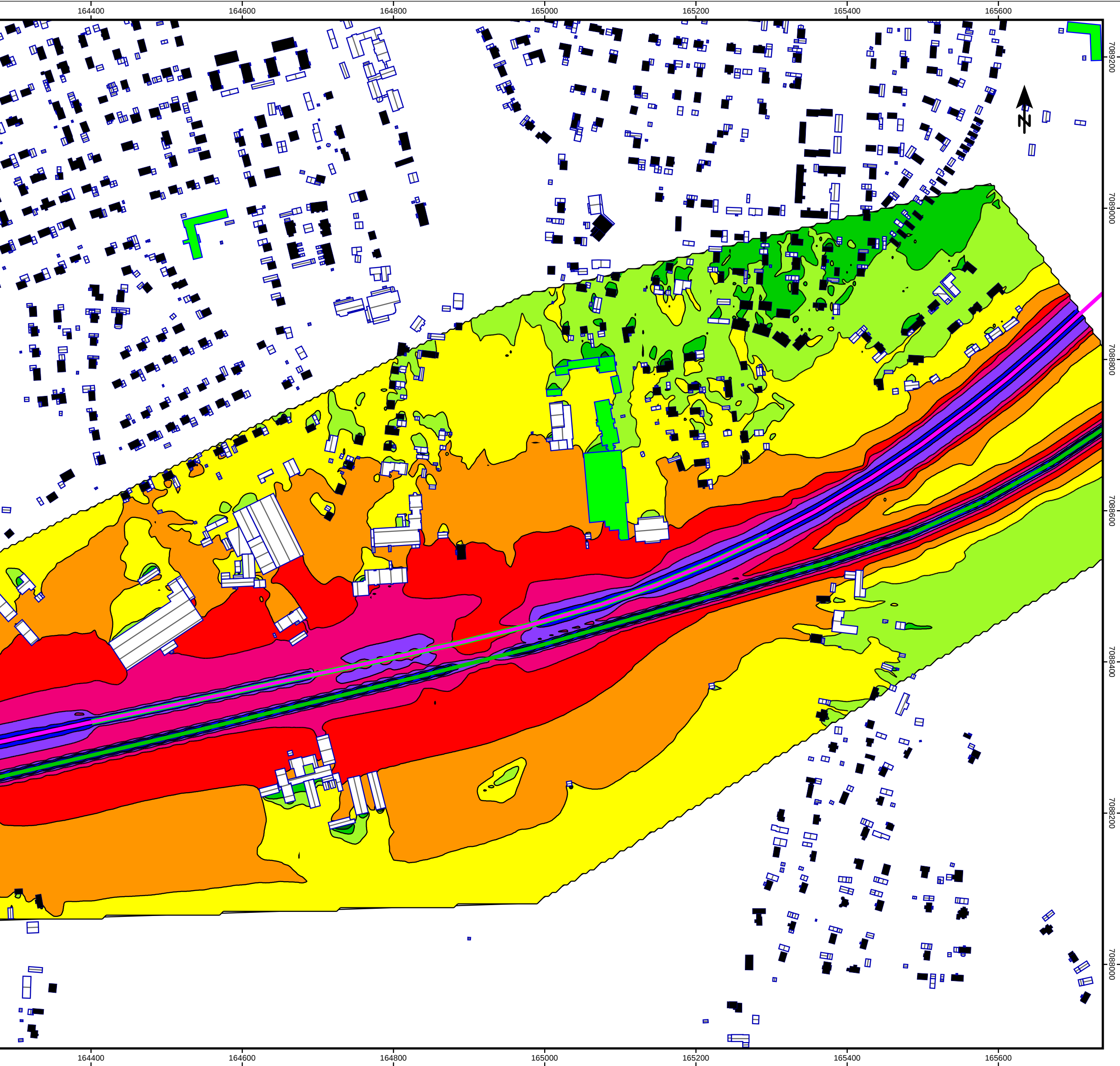
UTAN BULLERSKYDDSSKÄRM
