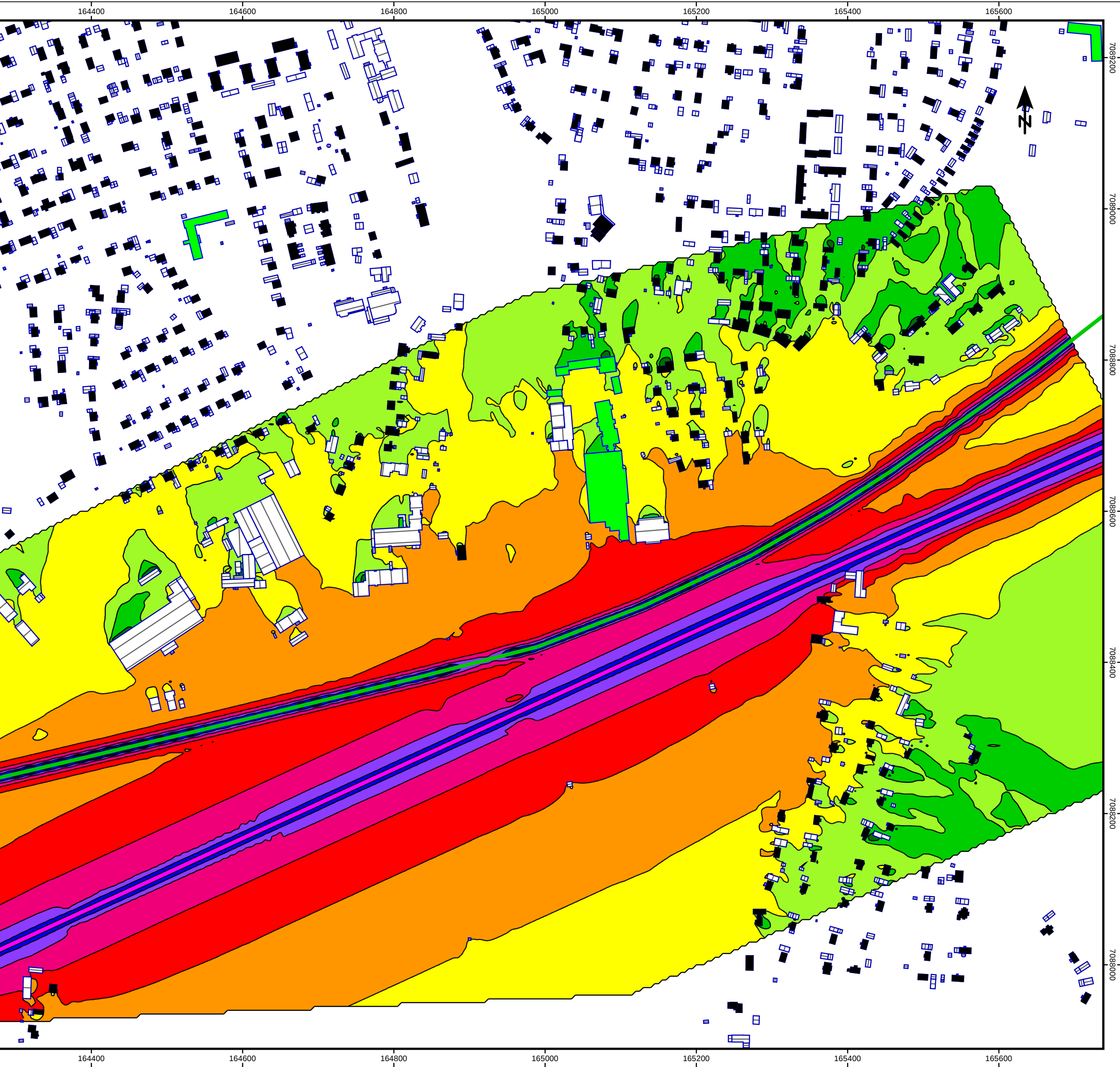
UTAN BULLERSKYDDSSKÄRM
