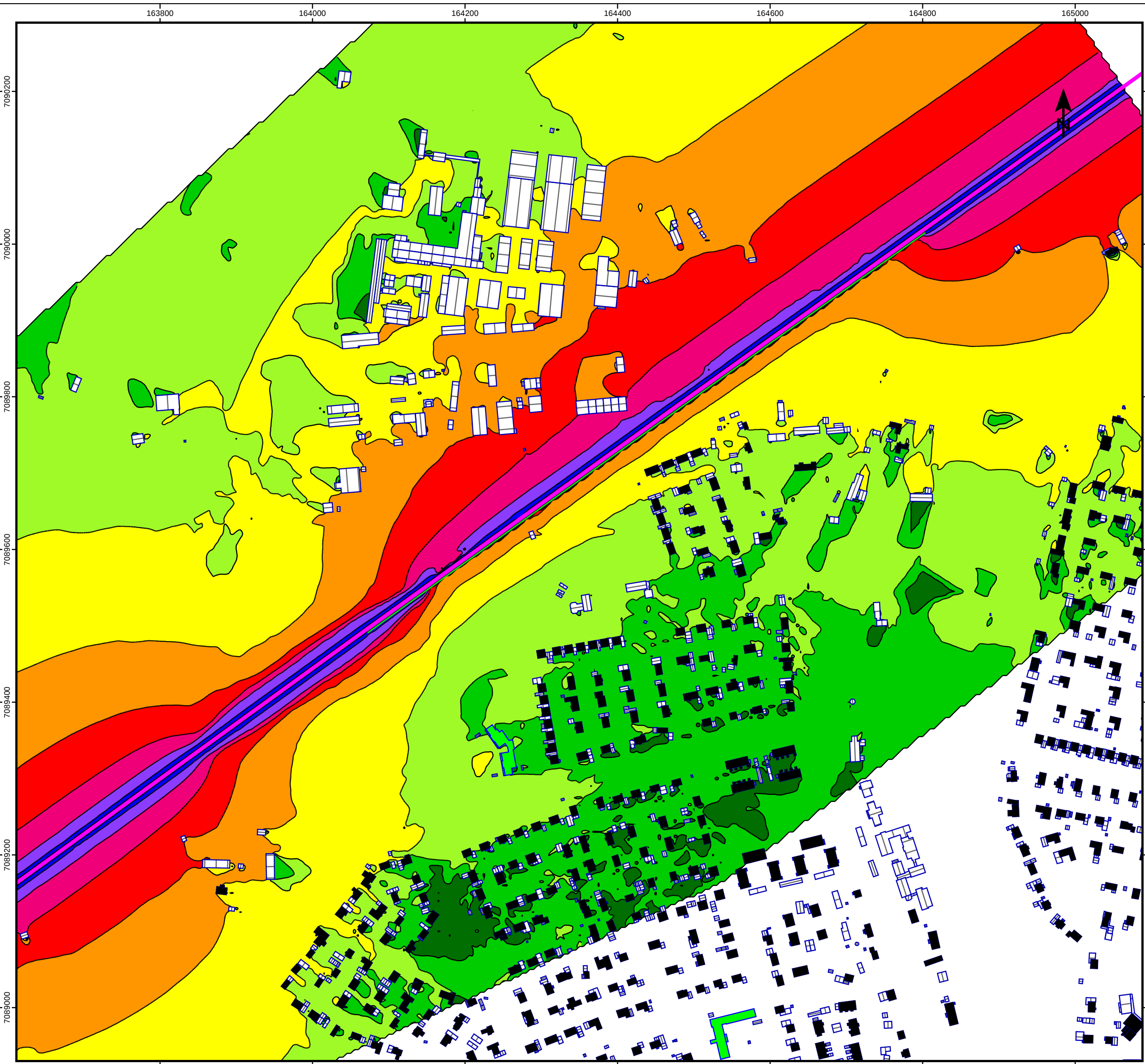
MED BULLERSKYDDSSKÄRM
