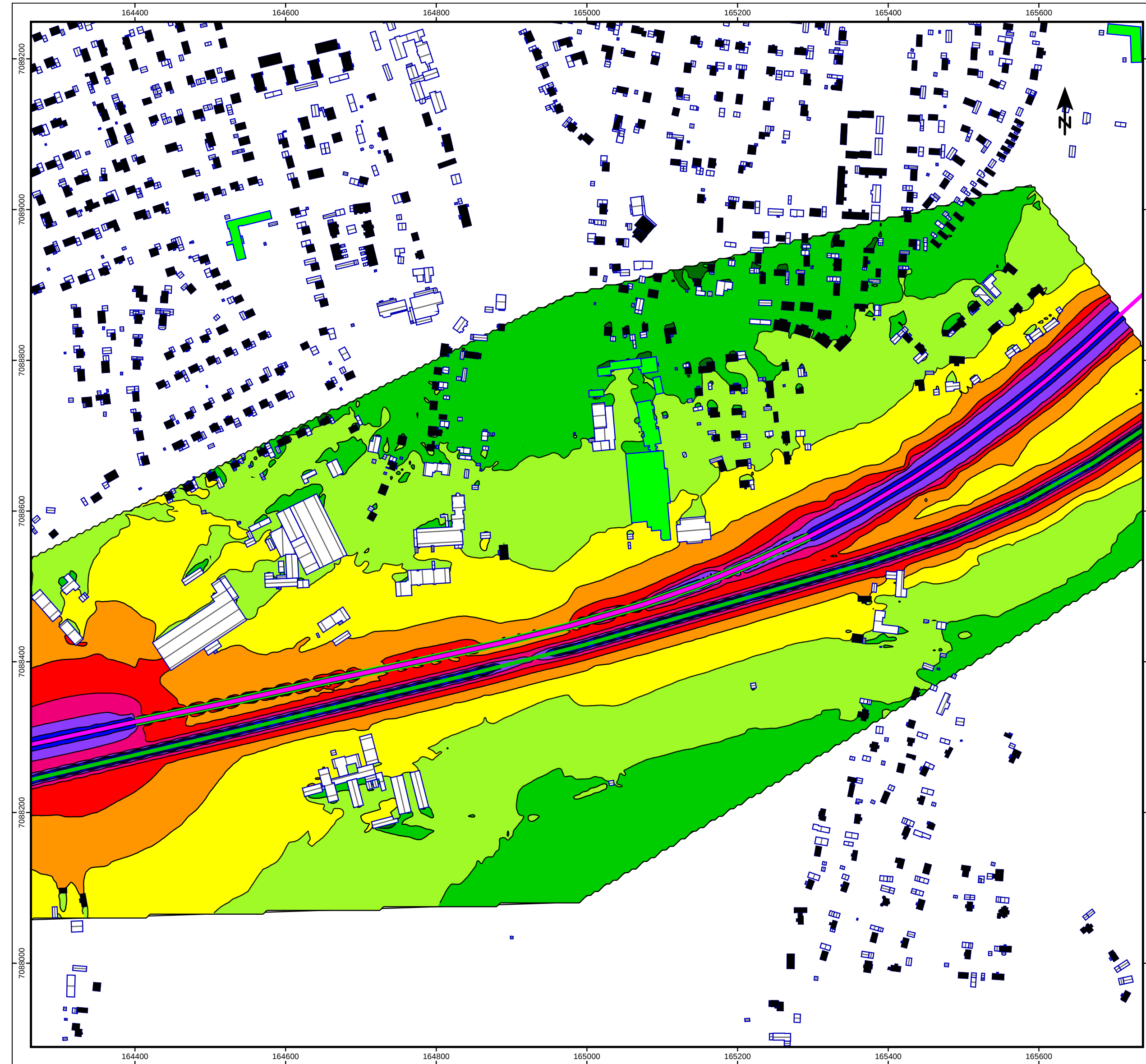
MED BULLERSKYDDSSKÄRM
