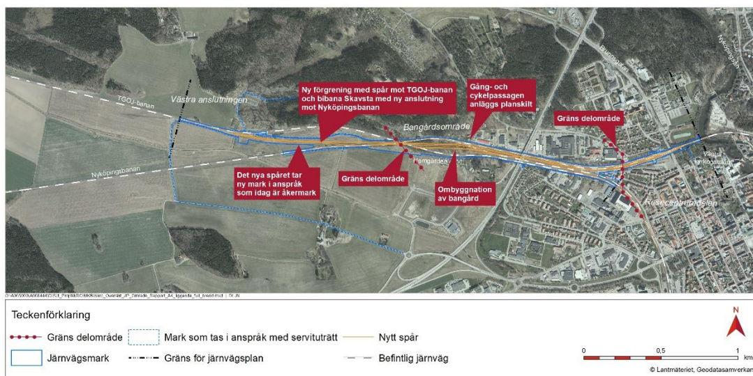
Figur 26. Översiktsskarta över järnvägsområdet och planerade åtgärder.
