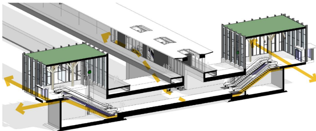
Figur 29. Principskiss över Centrala passagen med rörelseflöden markerade.
