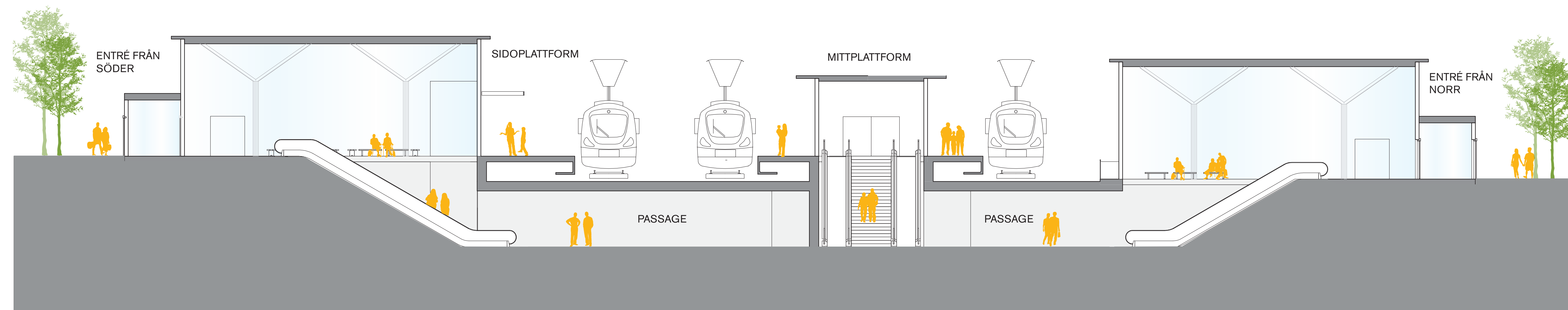
TVÄRSEKTION CENTRALA PASSAGEN, SKALA 1:100
