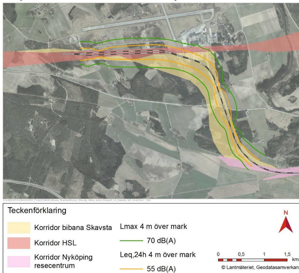
Figur 20. Bullerutredning ekvivalent och maximal nivå. OBS Linjen är fiktiv och har som enda syfte att vara underlag för bullerberäkningarna
