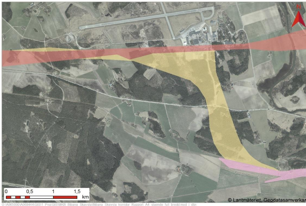
Figur 3 Avgränsning korridor för kort bibana med Skavsta station på bibanan, utredningsalternativ 1 (UA1).
