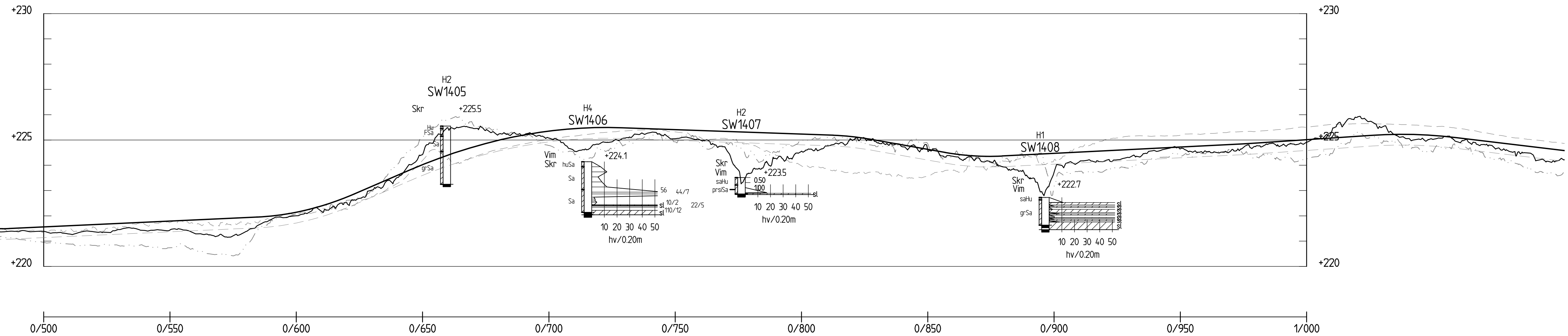
PROFIL H 1: 100 L 1:1000
