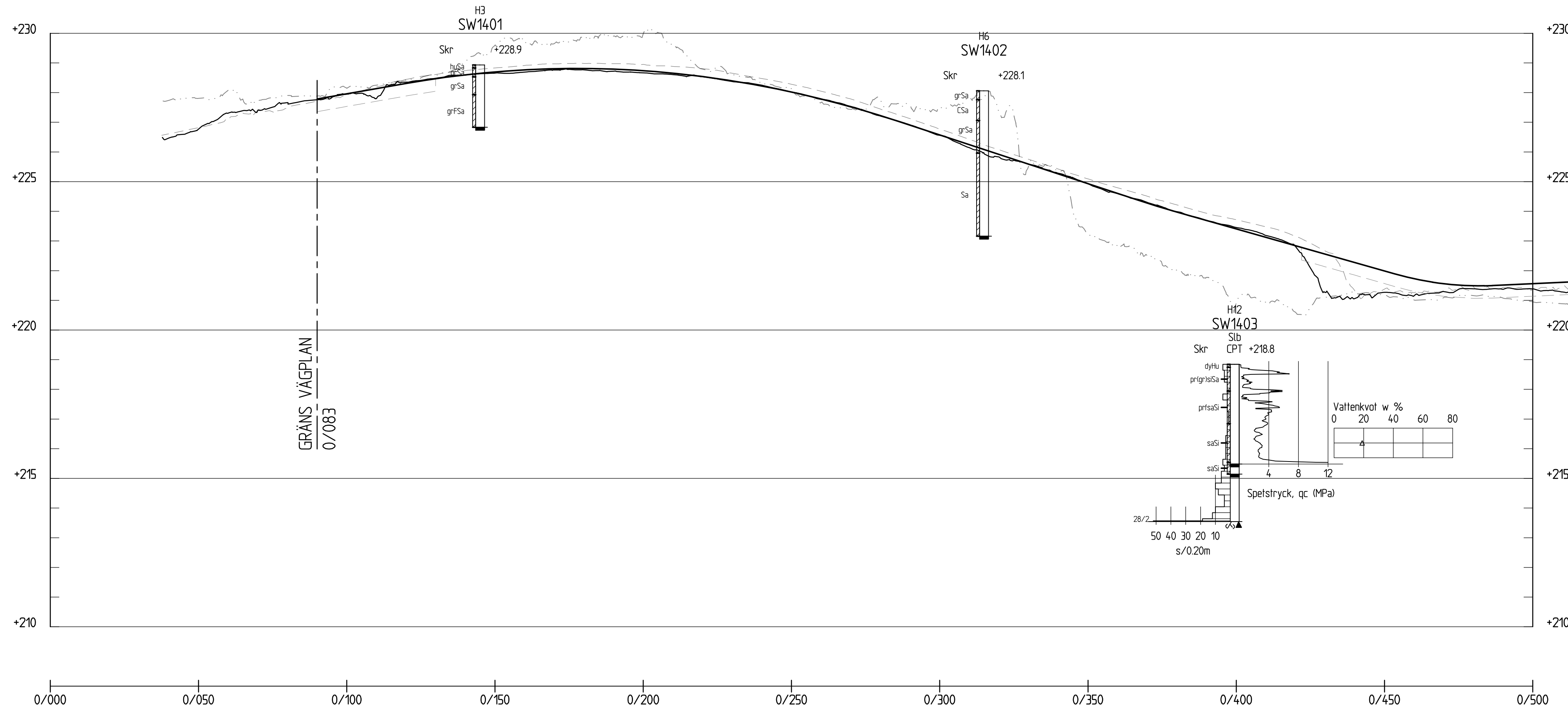
PROFIL H 1: 100 L 1:1000
