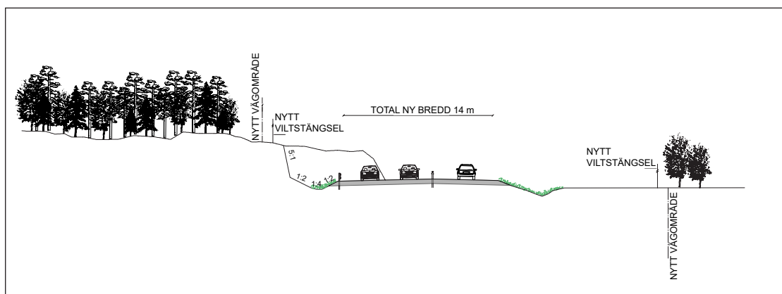
Bild 8. Princip för utformning av sidoområdet och anslutning till omgivande mark när vägen går på bank.
