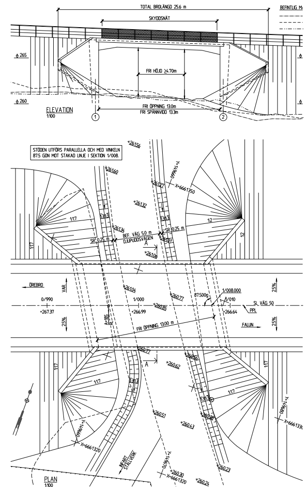
Utdrag ur förslagsritning bro över Djupuddsvägen (ej skalenlig)
