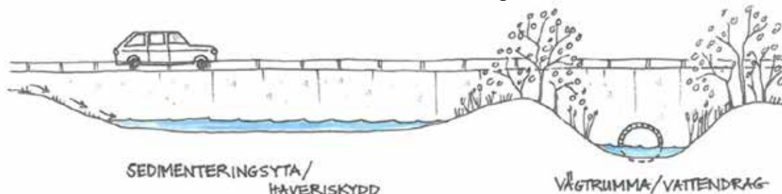
Illustration över principen för utformning på utsläppsdämme för sedimenteringsyta/haveriskydd. (Illustration Annika Persson)
