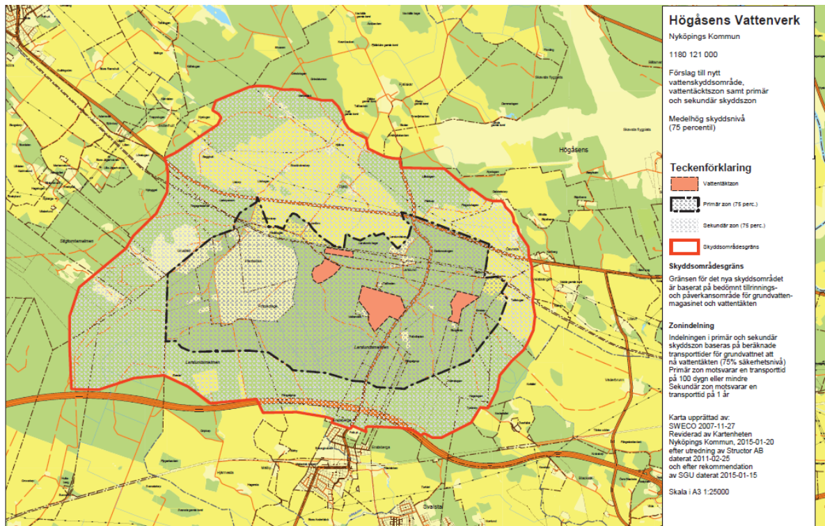
Figur 8. Skyddsområde Högsåns Vattenverk
