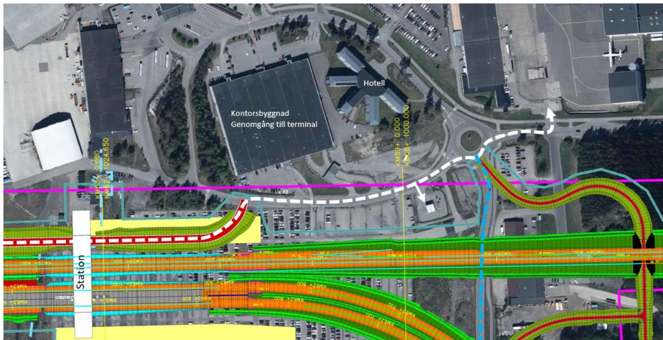
Figur 8. Översikt över stationsområdet och befintlig och framtida transportvägar till flygplats och bensinstation (blå resp. vit streckad linje).
