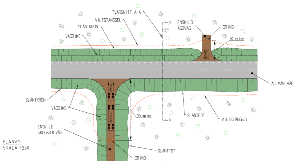
Figur 5.5 – Illustration över enskilda anslutningar med grind.
