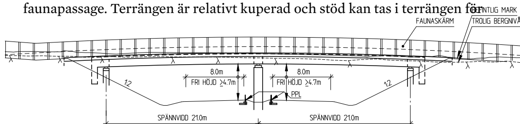
Figur 4.2.13. Förslagsskiss faunabro vid Södra Härene.
