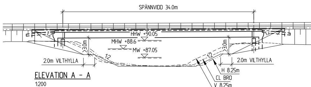
Figur 4.2.14. Förslagsskiss bro över Nossan med planerad vilthylla.
