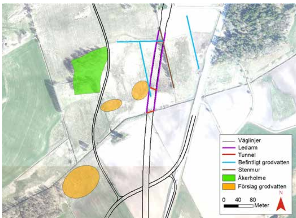
Figur 4.2.9 Förslag på nya grodvatten i höjd med Fötene (orangea områden). Markerad stenmur (brun) och åkerholmar (grönt) är viktiga övervintringsmiljöer. Svarta linjer markerar nya vägar. Lila linjer visar ledarmar som kan hindra groddjur från att ta sig upp på väg E20.
