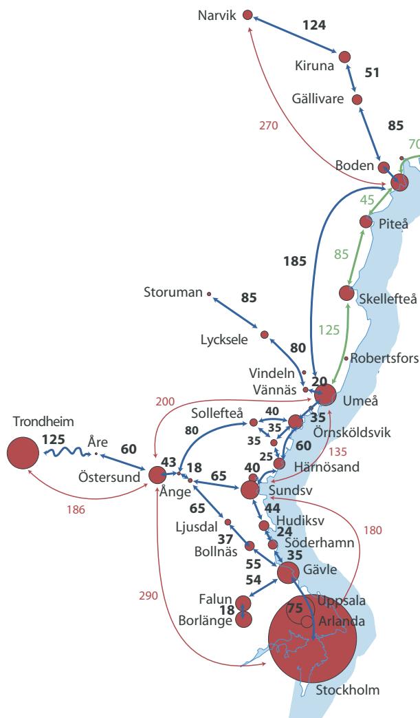
Figur 4.2b: Restidsavstånd vid ett nollalternativ med Botniabanan utbyggd. Källa: ÅF Infraplan.
