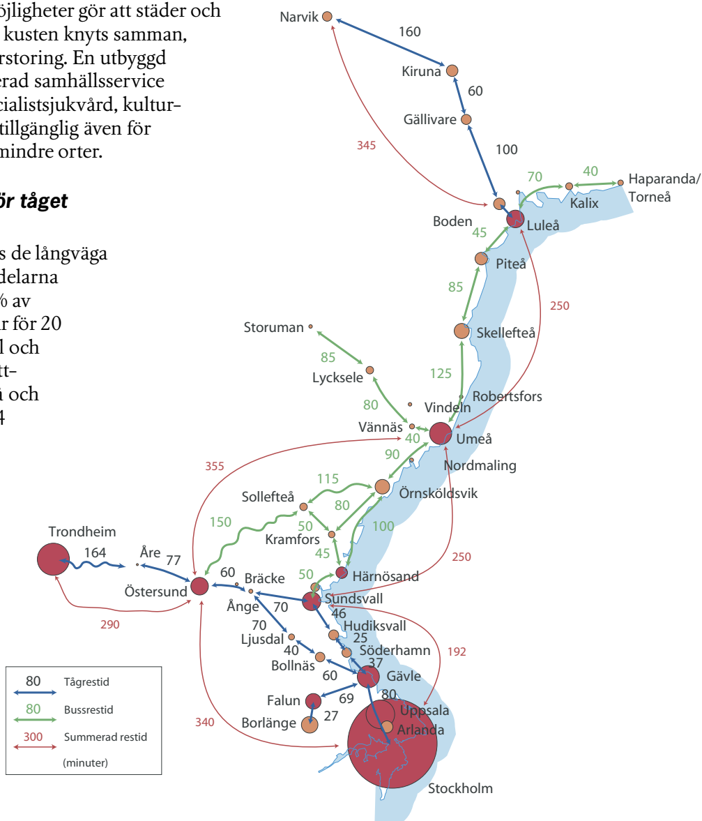
Figur 4.2a: Restidsavstånd med dagens transportmedel. Källa: ÅF Infraplan.
