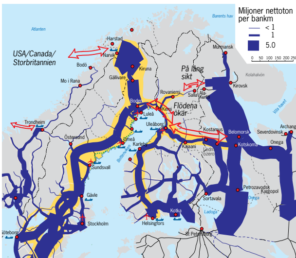
Figur 4.1: Godsvolym i Norden och Ryssland. Källa ÅF Infraplan.
