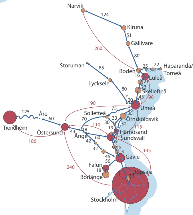
Figur 4.2c: Restidsavstånd med Botniabanan och Norrbotniabanan utbyggda. Även omfattande upprustning av exempelvis Ådalsbanan och Ostkustbanan ingår i denna bild. Källa: ÅF Infraplan.
