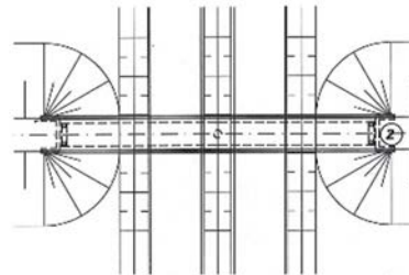
Principförslag för bro över 2+2-väg i plan.
