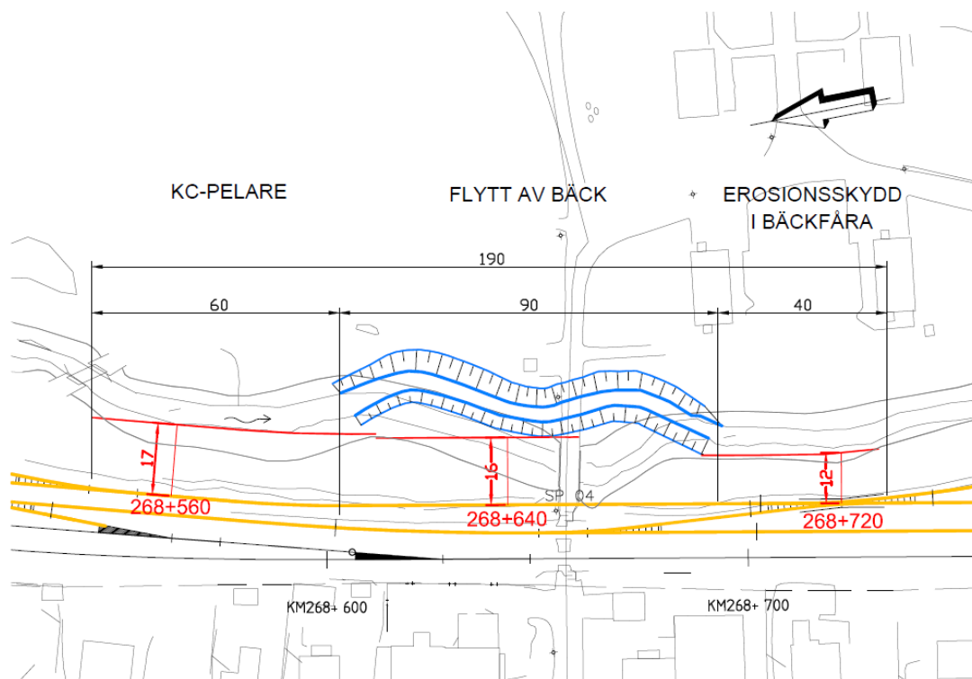
Figur 13 Stabiliserande åtgärder
