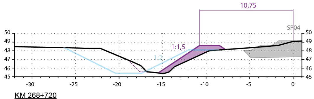
Figur 14 Lila område visar föreslaget erosionsskydd. Alternativet är att flytta bäcken till den blå linjen som både blir dyrare och är sämre för vattenmiljön.
