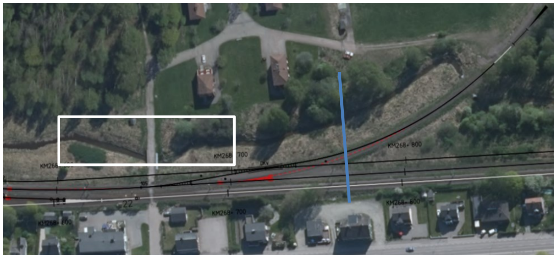
Figur 12 Röda linjer visar spår och växlar som tas bort eller flyttas. Svarta linjer är nya eller flyttade spår och växlar. Grått visar det som inte påverkas. Blå linje visar järnvägsplanens slut. Övriga spår ligger på Gruvöns fastighet. Vit ram visar det område som berörs av omgrävning av bäcken.
