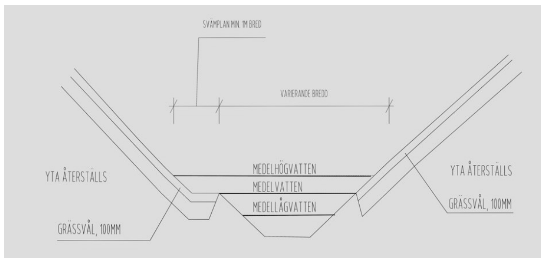
Figur 15 Förslag på utformning av ny bäckfåra (bild från Naturcentrum). Översvämningsyta föreslås på ena sidan (plan yta till väster i bilden).
