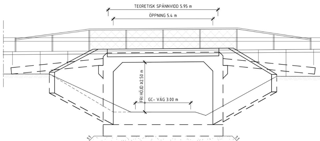
Figur 5.1.2–1 Förslagsskiss över broutformningen.
