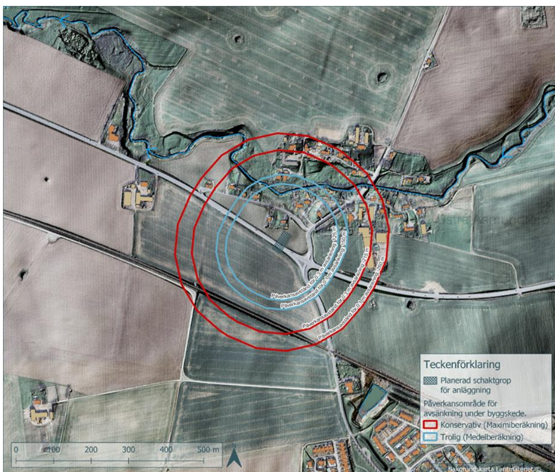
Figur 6.3.7–1. Avsänkningens utbredning i det undre magasinet vid en temporär avsänkning under byggskedet. I figuren illustreras fyra olika påverkansområden. Röda områden avser de mest konservativa beräkningarna och visar påverkansområden där avsänkning är större än 0,1 samt 0,3 m från ostörda grundvattennivåer. Blå områden avser de troligaste beräkningarna och visar på motsvarande sätt påverkansområden där avsänkning är större än 0,1 samt 0,3 m från ostörda grundvattennivåer.
