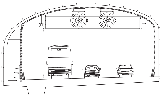
Figur 27 Exempel på en tvärsektion av ett av tunnelrören.
