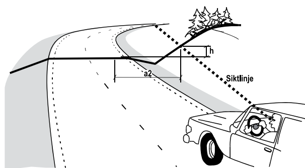
Figur 26 Principskiss sikt längd.
