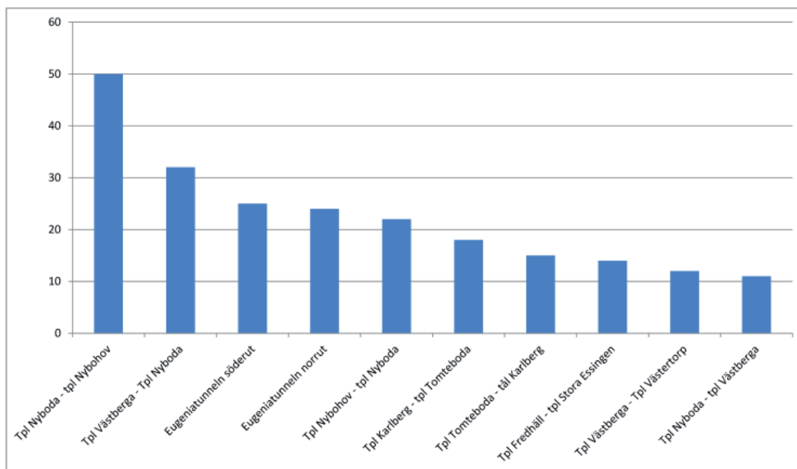
Figur 9 E4 genom Stockholm, incidenter 2004-2009. De tio mest belastade vägsträckorna. Antal incidenter per miljon fordonsskilometer.
