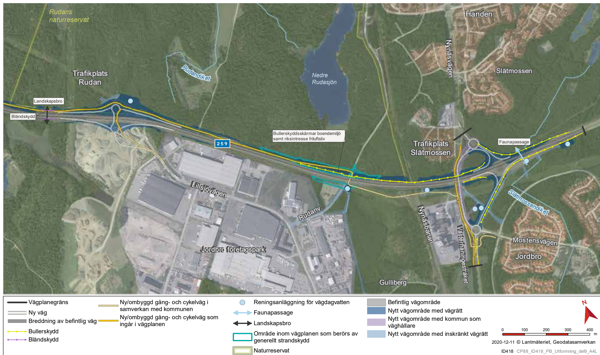
Figur 3.36 Väg 259 samt gång- och cykelväg i trafikplats Rudan och trafikplats Slätmosse.
