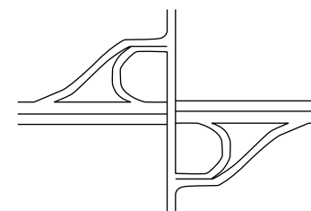
Trafikplats med klöverramper. Avfartsrampöglorna är formade som klöverblad.
