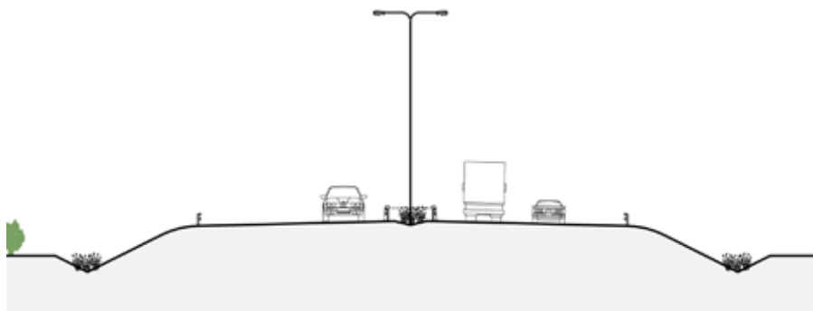
Figur 3.6 Väg 259 med tre körfält i vardera riktningen.
