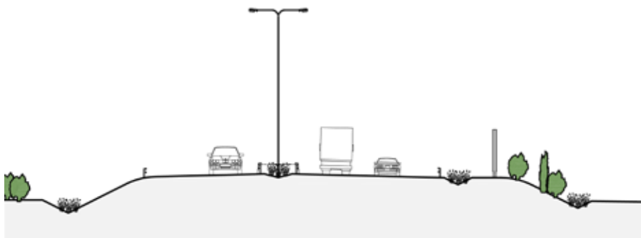
Figur 3.8 Väg 259 med bullerskyddskärm.
