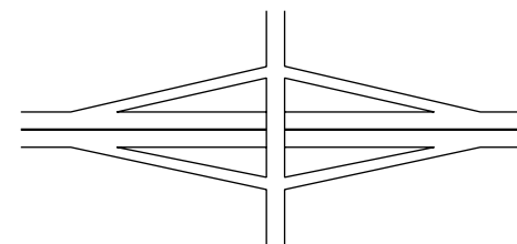
Trafikplats med ruterramper. Parallella på- och avfartsramper ger trafikplatsen en ruterform.
