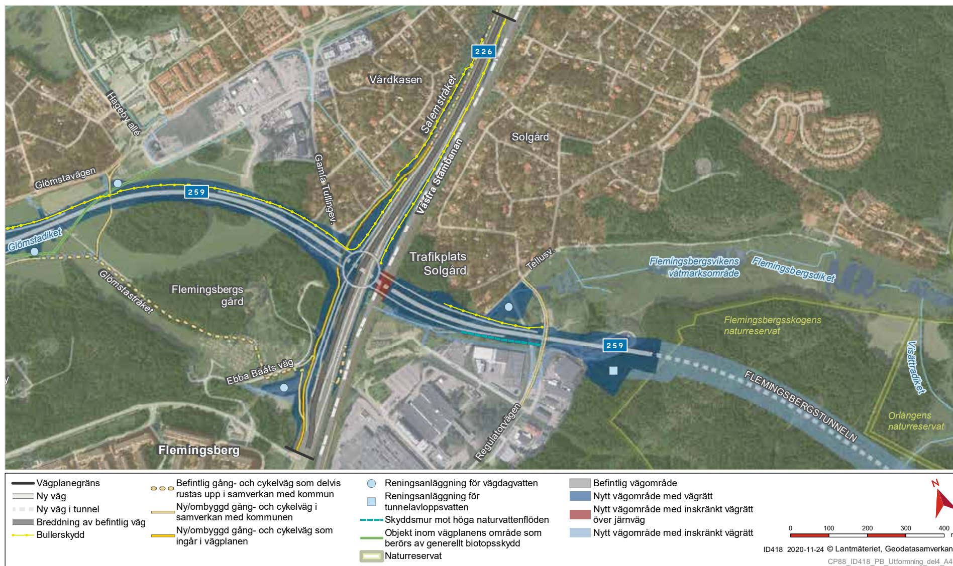
Figur 3.22 Väg 259 och väg 226 vid trafikplats Solgård samt väg 259 vid Flemingsbergstunnelns västra mynning. Gång- och cykelväg i Glömstadalen, längs med Glömstavägen och väg 226.
