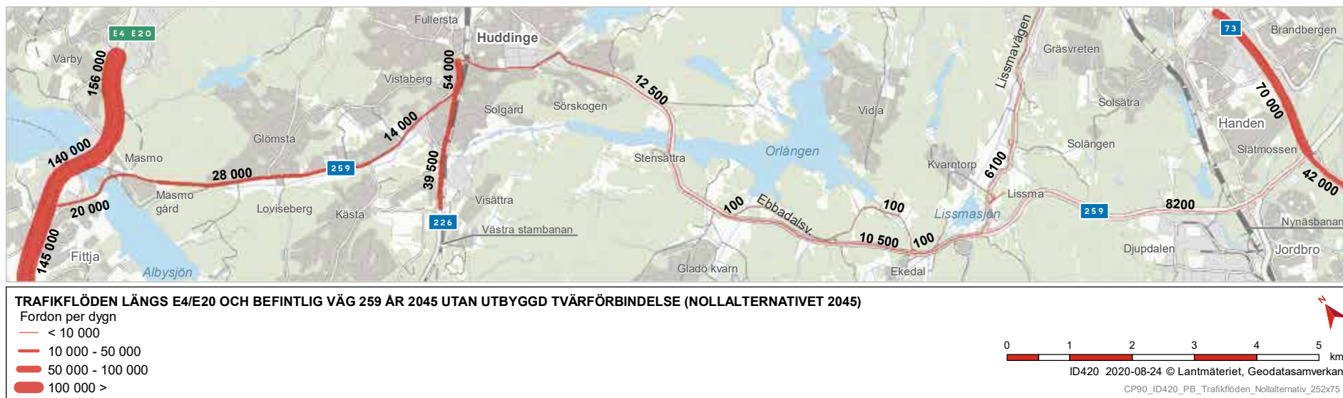
Figur 2.2 Trafikflöden under ett årsmedeldygn längs E4/E20 och befintlig väg 259 år 2045.
