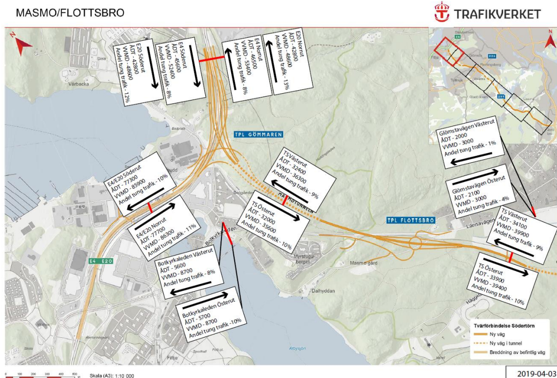
Figur 4. Flöden Gömmaren/Flottsbro för årsmedeldygn (ÅDT), vintervardagsmedeldygn (VMD) samt andel tung trafik.
