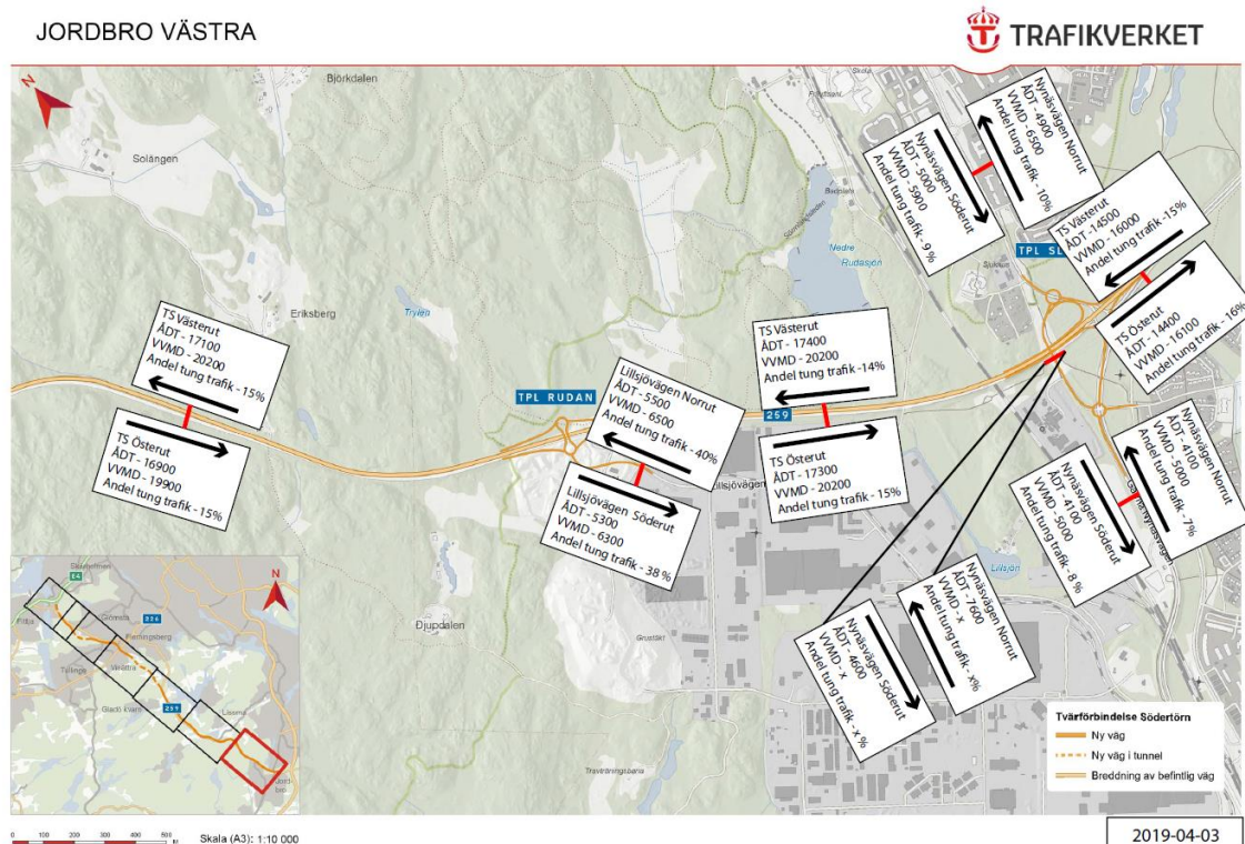
Figur 9. Flöden Jordbro (Rudan/Slätmossen) för årsmedeldygn /ÅDT), vintervardagsmedeldygn (VVMD) samt andel tung trafik.
