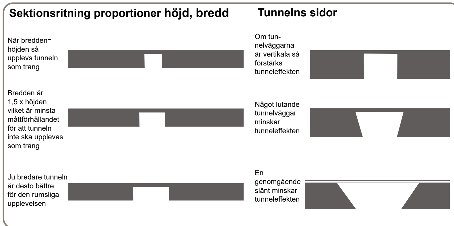
Figur 3 och 4: Principer för utformning av gång- och cykelpassager (Vägverket, 2001)
