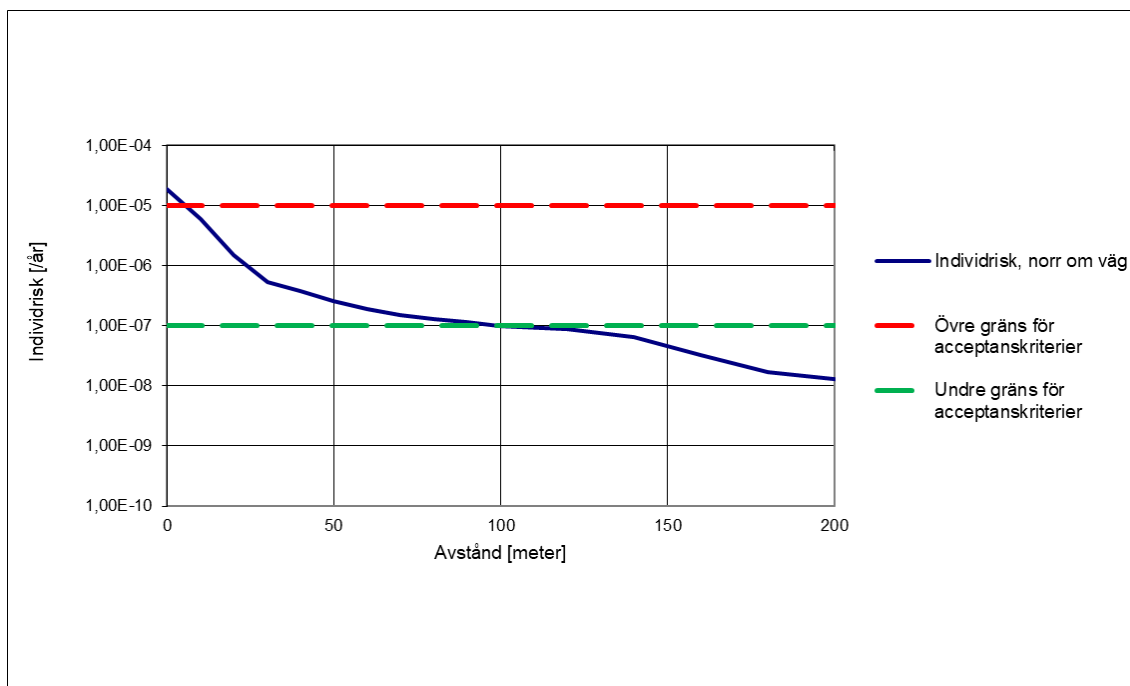
Figur 80. Individerisk TS vägavsnitt 9 med åtgärder, norr om väg
