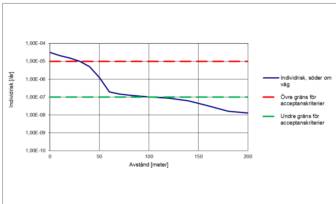
Figur 48. Individrisk TS vägavsnitt 10 utan åtgärder, söder om väg
