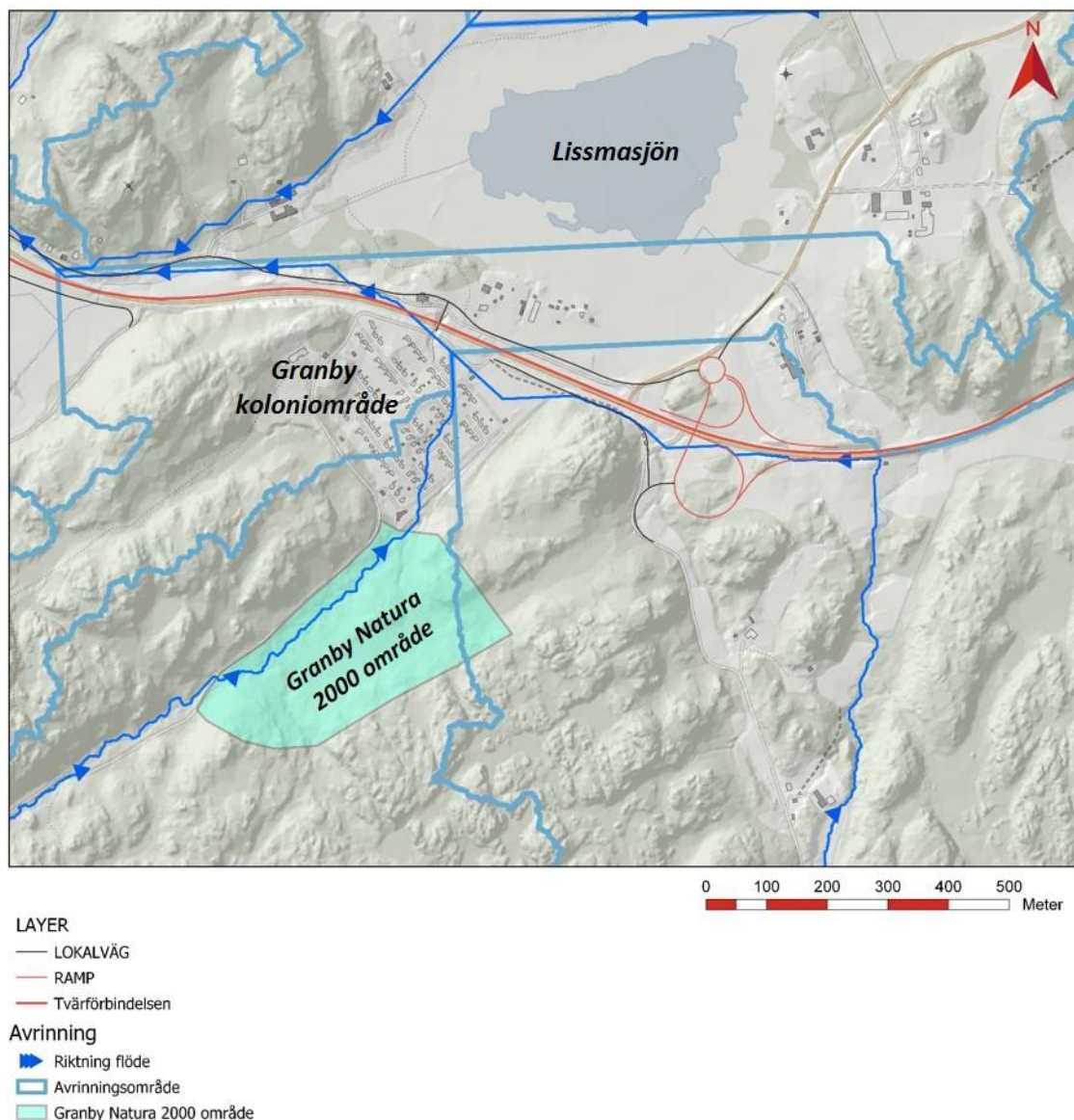
Figur 2. Avrinningsområden och flödesriktningsberäkningar kring Granby och Lissma. Beräkningarna är gjorda utifrån en höjdmödel med 1.5 x 1.5 m pixlar. Flödet är från söder mot nord-nordväst.
