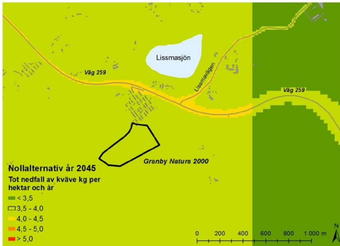
Figur 9. Beräknad total deposition av kväve för nollalternativet 2045. Jämfört med nuläget minskar depositionen i 0-alternativet. Analysen består av flera olika beräkningar med olika noggrannhet och rumslig avgränsning, som sedan är överlagrade på varandra. Detta syns som skillnad i pixelstorlek, samt gränsen mellan ljusgrönt och mörkgrönt.
