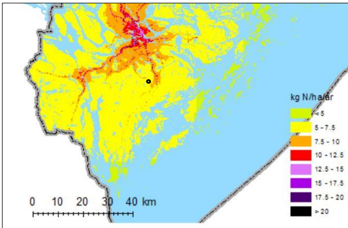
Figur 6. Beräknad total deposition av oorganiskt kväve för år 2015. Bild tagen från Stockholms Länsstyrelse rapport "Kvävedeposition i Stockholms län år 2015", Fakta 2017:4. Grön prick markerar ungefärlig plats för Granby natura 2000 område.
