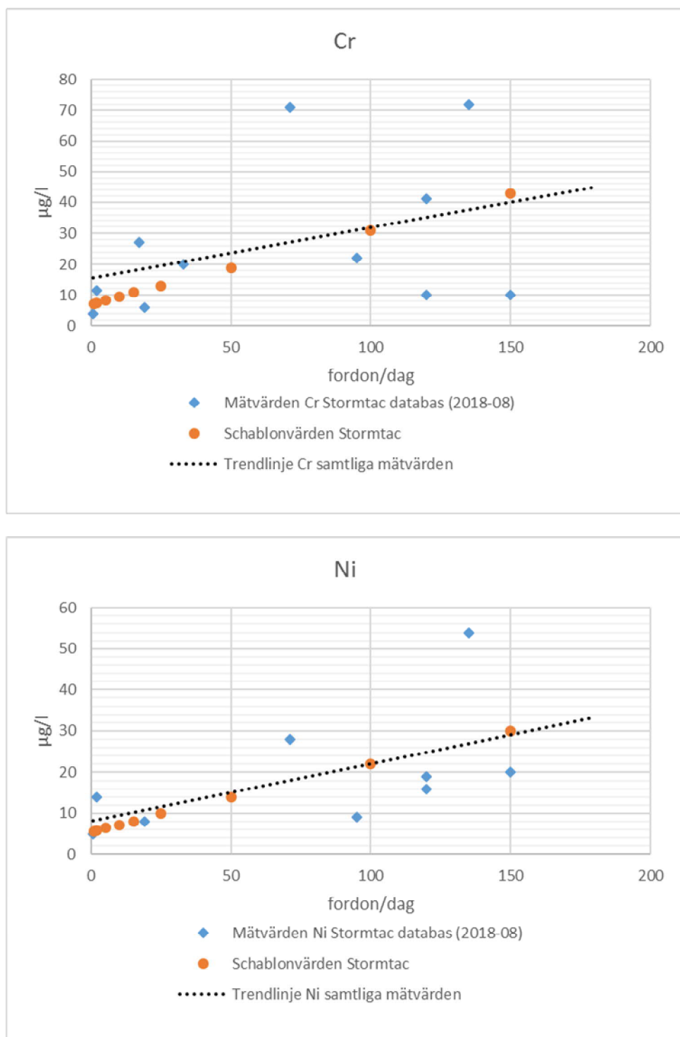
Figur 4. Haltvärden från Stormtac:s databas, samtliga värden där trafikintensitet är angivet (augusti 2018) för krom (Cr) och nickel (Ni) samt trendlinjer baserade på samtliga data, och Schablonvärden från Stormtac.
