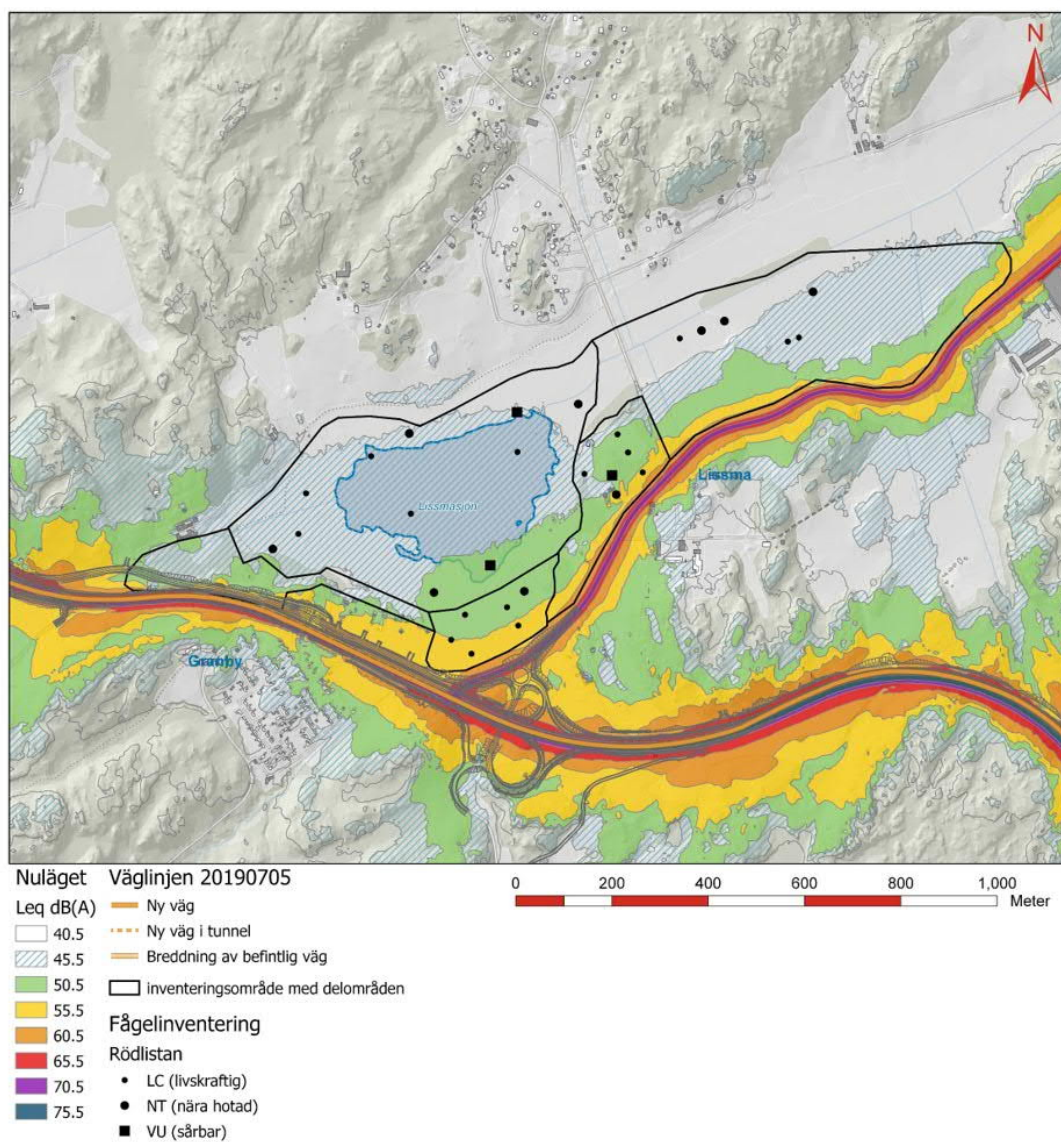
Figur 29. Bullerutbredning, nuläge.
