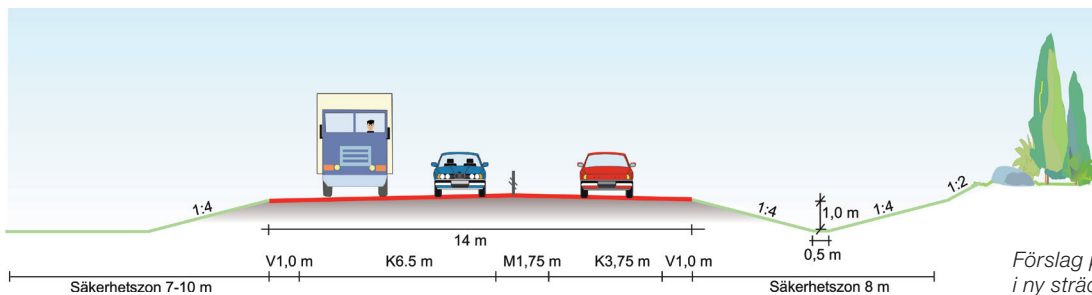
Förslag på sektion 1+1 i ny sträckning
