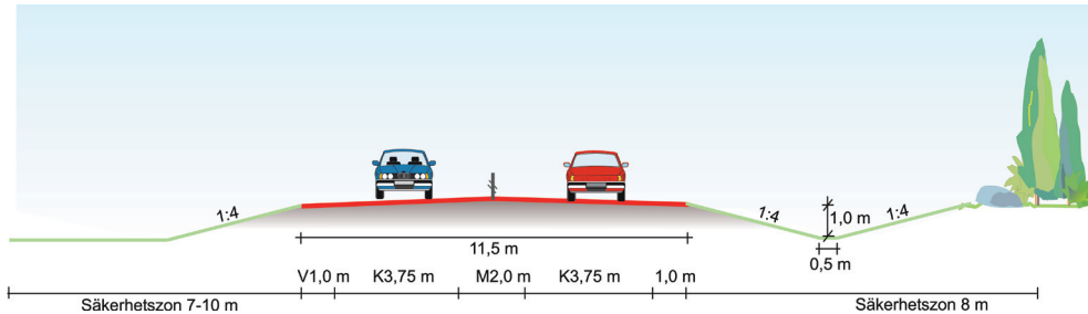
Förslag på sektion 1+1 i ny sträckning
