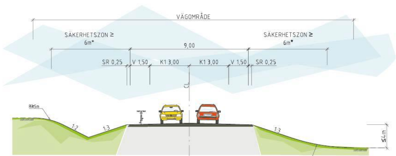
Figur 4.2.1.4 Typsektion lokalväg 2755.
