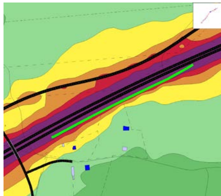
Figur 23: Vägnära vall nr 5. Ekvivalent ljudnivå, 2m över mark: Efter åtgärd
