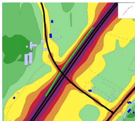
Figur 17: Vägnära vall nr 2. Ekvivalent ljudnivå, 2m över mark: Efter åtgärd
