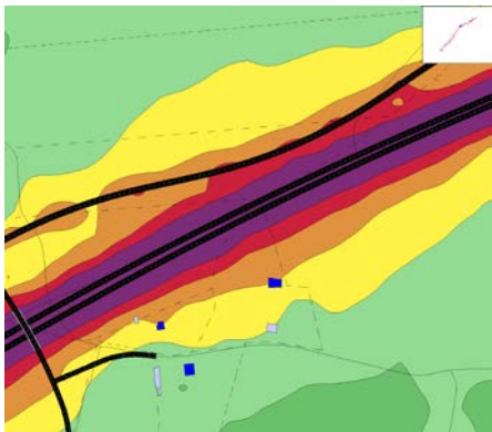
Figur 22: Vägnära vall nr 5. Ekvivalent ljudnivå, 2m över mark: Före åtgärd
