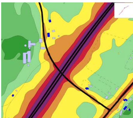
Figur 16: Vägnära vall nr 2. Ekvivalent ljudnivå, 2m över mark: Före åtgärd
