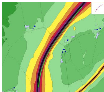
Figur 15: Vägnära vall nr 1. Ekvivalent ljudnivå, 2m över mark: Efter åtgärd
