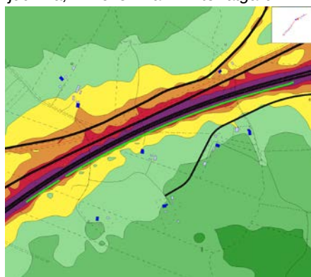
Figur 19: Vägnära vall nr 3. Ekvivalent ljudnivå, 2m över mark: Efter åtgärd
