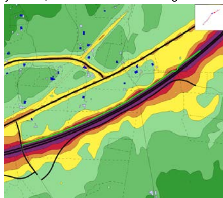
Figur 21: Vägnära vall nr 4. Ekvivalent ljudnivå, 2m över mark: Efter åtgärd
