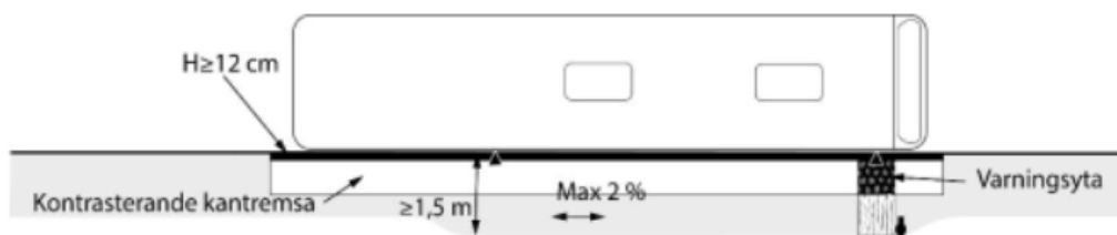
Figur 16. Principutformning av plattformstyp 4.
