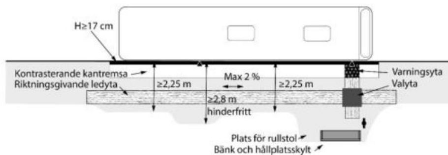
Figur 17. Principutformning av plattformstyp 2.
