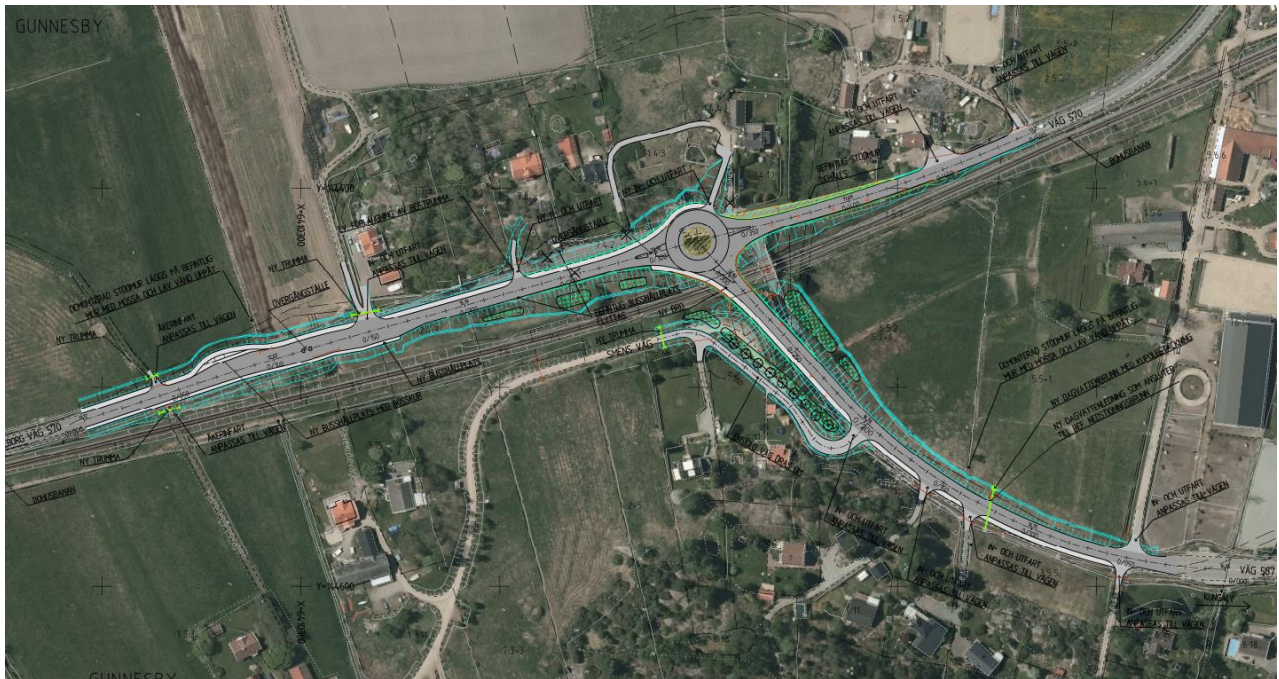
Figur 23. Vägförslag med ny bro och cirkulationsplats.
