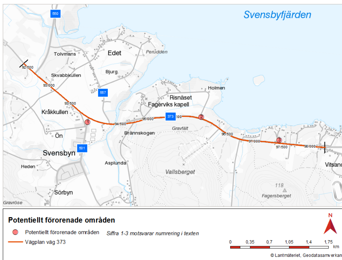
Figur 4.8.1. Potentiellt förorenade fastigheter i närområdet till vägplaneområdet för väg 373.
