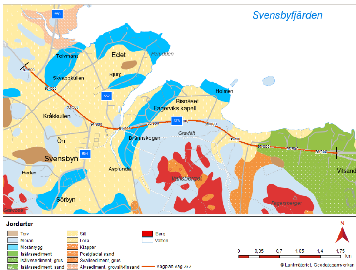
Figur 2.6.1. Jordarter i området.
