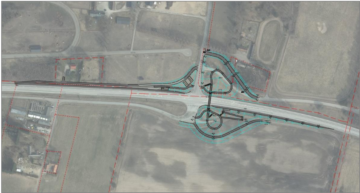
Figur 34 - Alternativ med gång- och cykelpassage över väg 11, på östra sidan.
