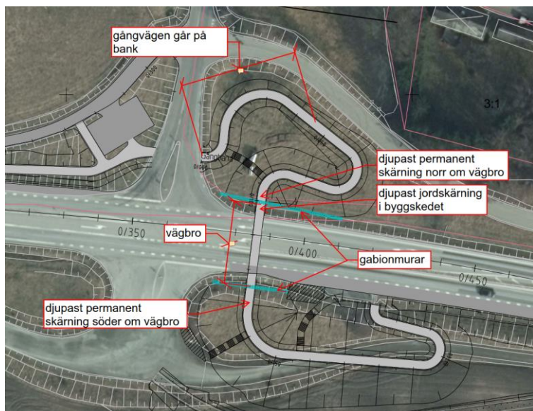
Figur 25 - Aktuell delsträcka med förslag till projekterad anläggning.
