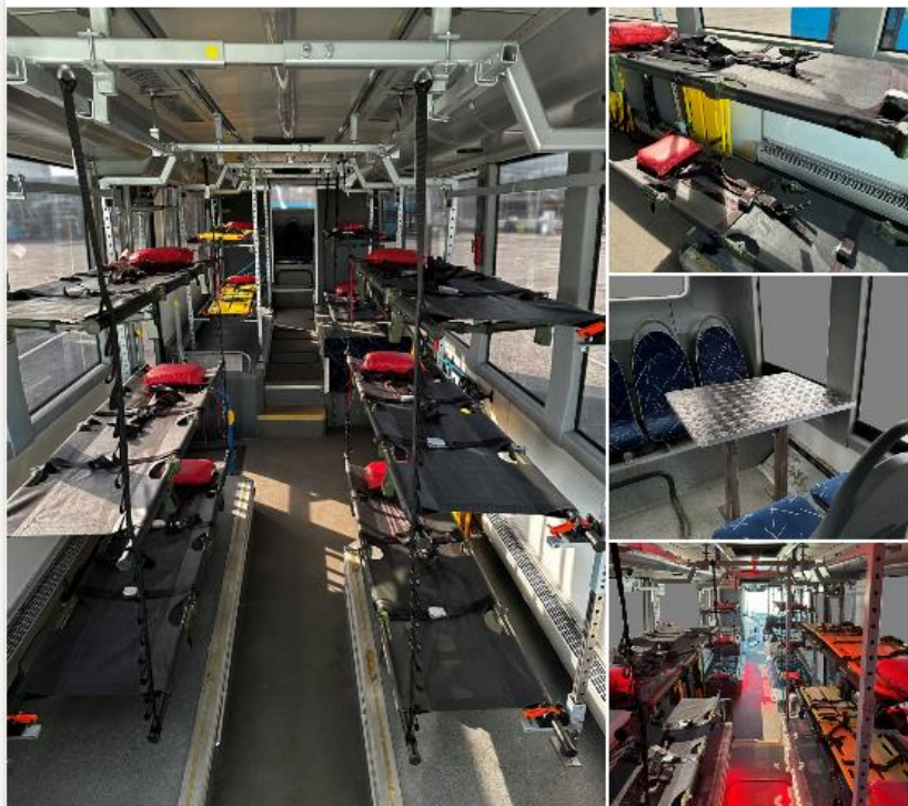
Lösning med konvertibel citybuss VGR/Västtrafik
