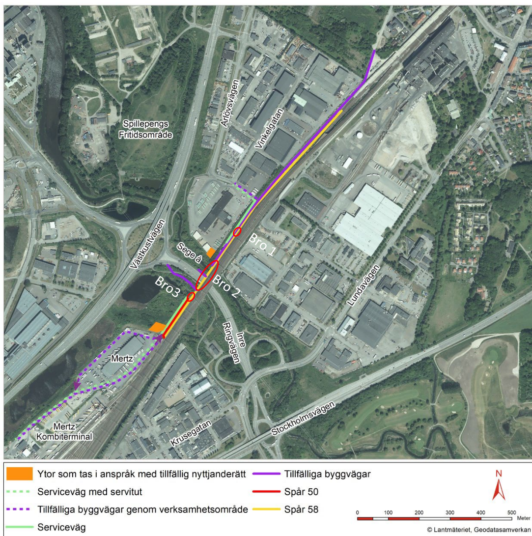
Figur 4.4. Översiktlig utformning av driftskedet och byggskedet.
